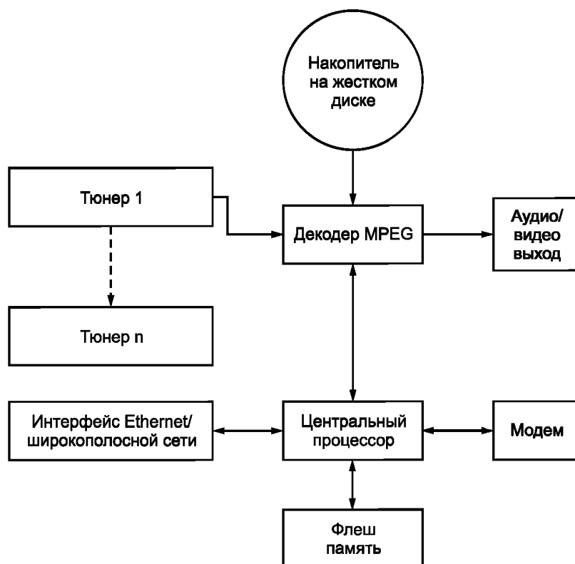
Рисунок D.1 — Блок-схема основных функциональных частей РЦТ
