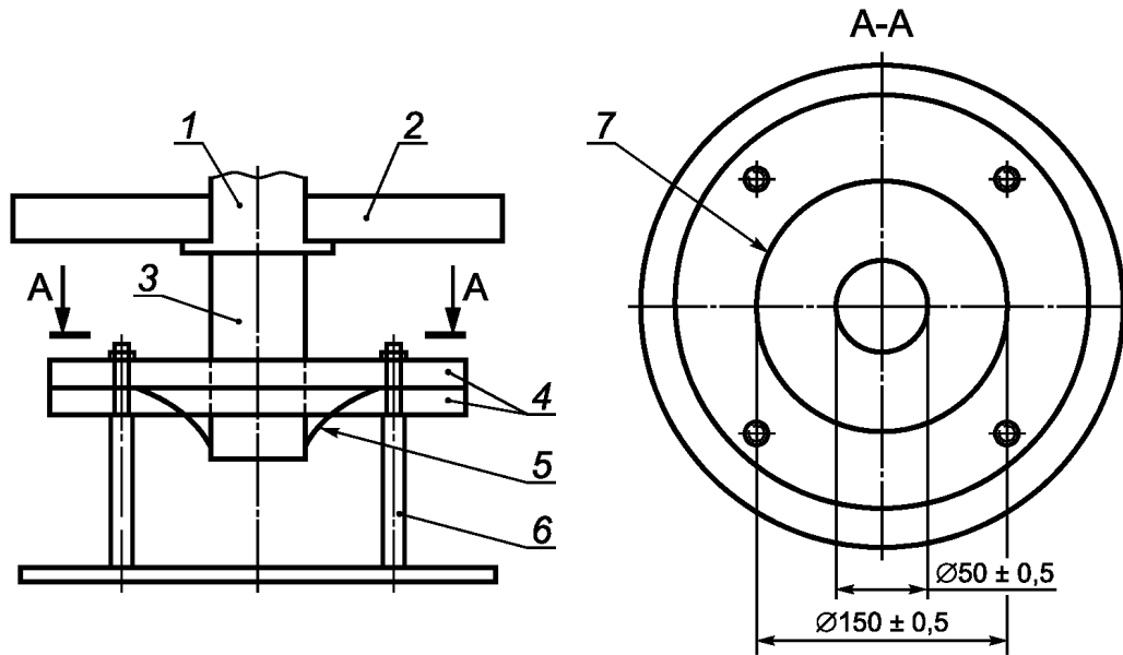
1 — датчик сжимающей нагрузки; 2 — поперечина; 3 — плунжер; 4 — зажимные кольца; 5 — образец; 6 — несущая рама или форма CBR; 7 — скругленные внутренние кромки Рисунок Е.2 — Пример зажимного приспособления
