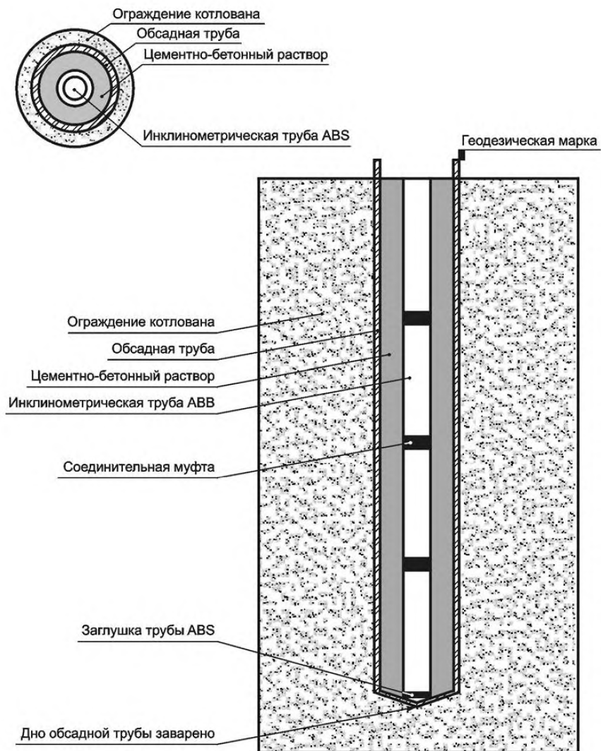
Рисунок Д.1 — Схема инклинометрической наблюдательной скважины
