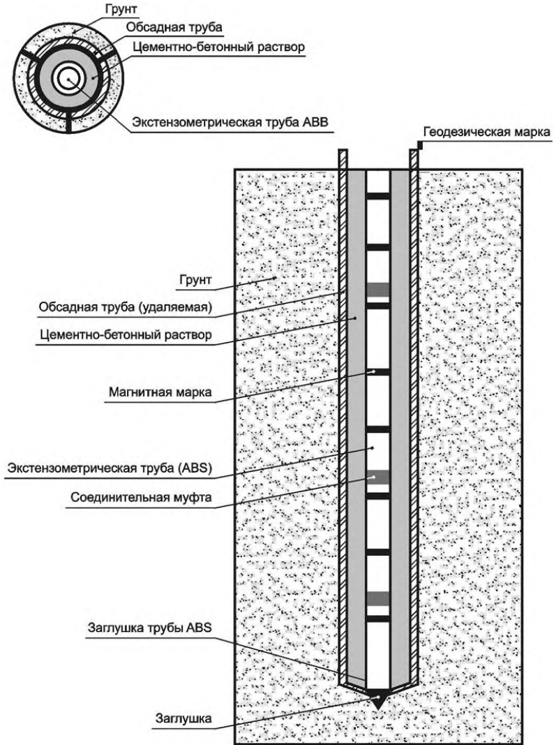
Рисунок Д.2 — Схема экстензометрической наблюдательной скважины
