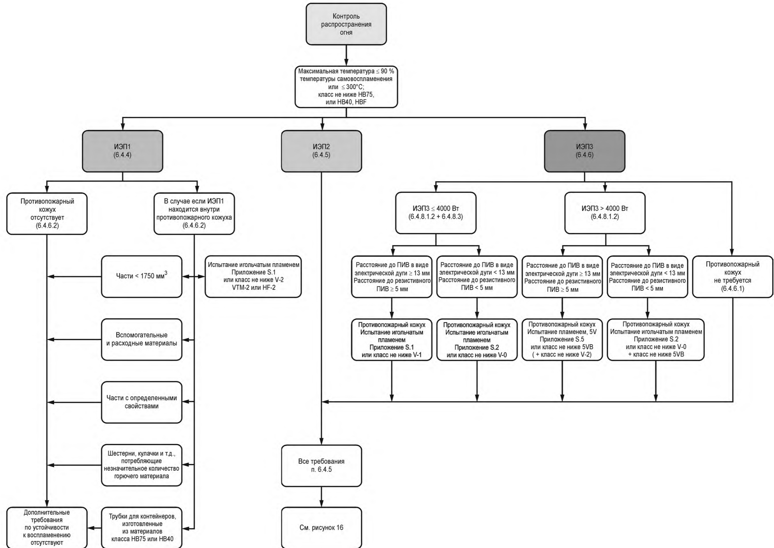
Рисунок 15 — Сводная информация по контролю распространения огня
