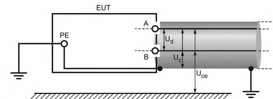
Локальное заземление (бетонный пол, металлический трубопровод и т.д.) Интерфейс сдвоенного провода – экранированный кабель
