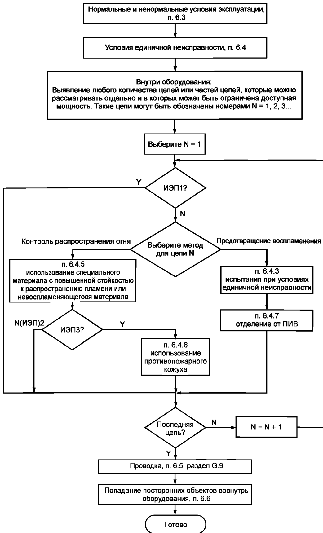
Рисунок 13 — Блок-схема разделов, касающихся возгораний
