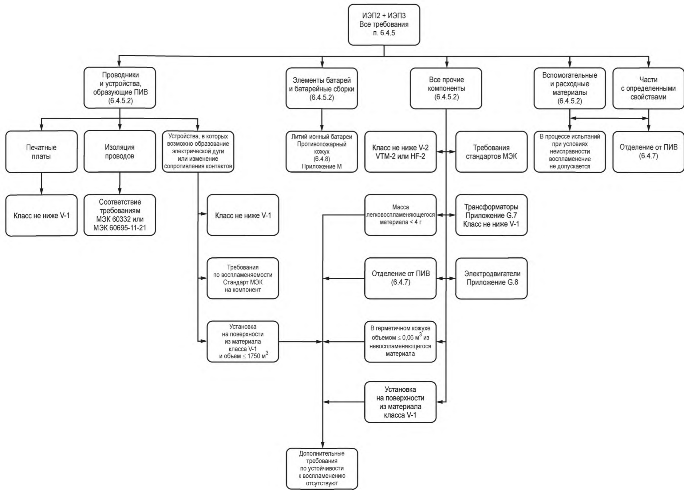
Рисунок 16 — Сводная информация по контролю распространения огня (2)
