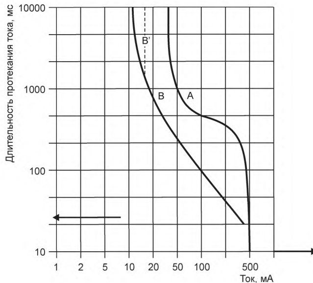
Рисунок 26 — Кривые предельного тока
