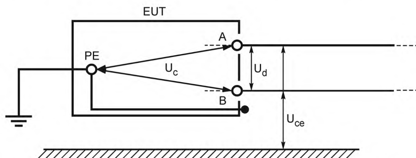
Локальное заземление (бетонный пол, металлический трубопровод и т.д.) Интерфейс сдвоенного провода – незэкранированный кабель
