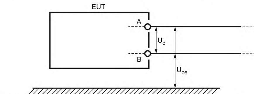
Локальное заземление (бетонный пол, металлический трубопровод и т.д.) Интерфейс сдвоенного провода – без заземления
