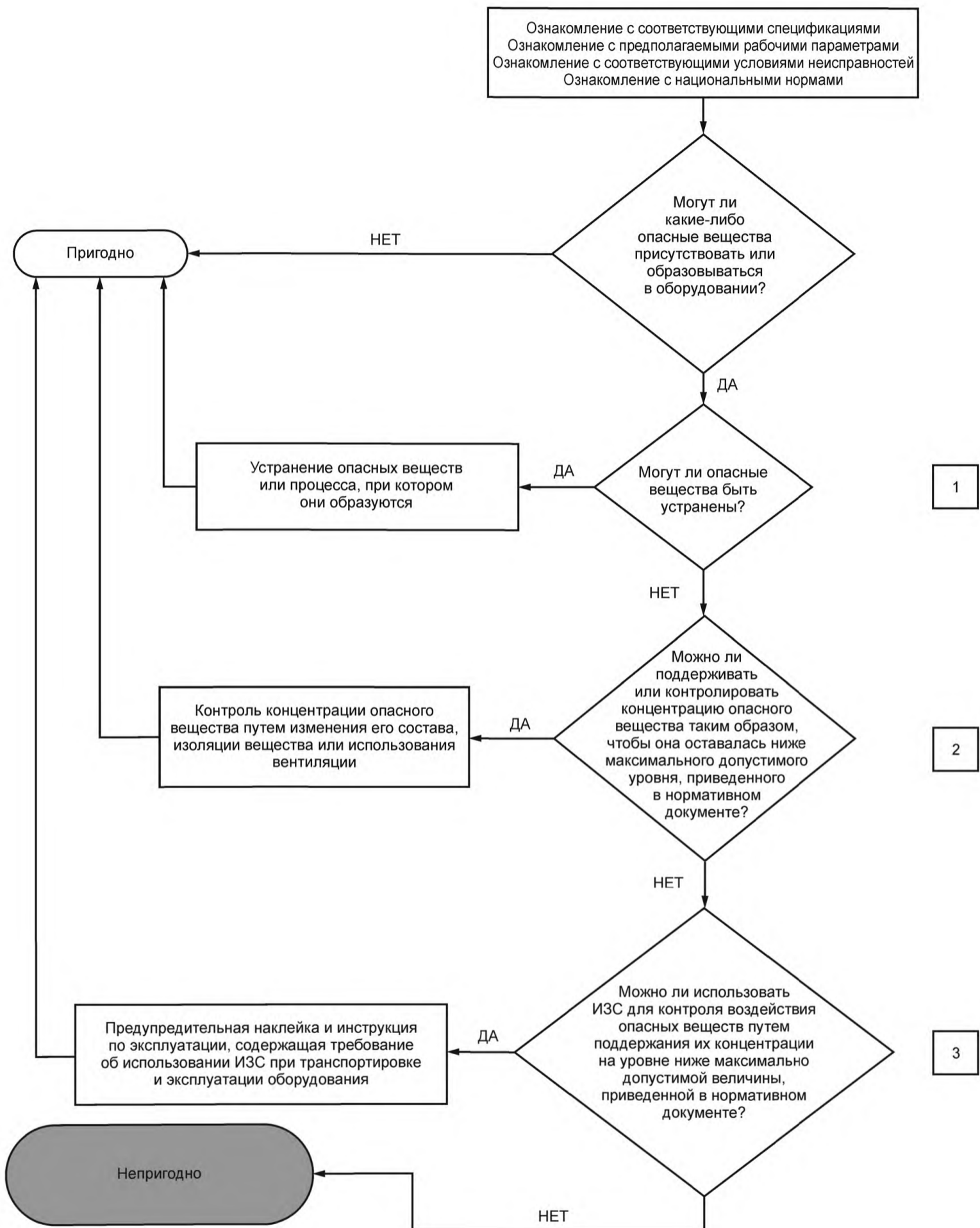
Рисунок 18 — Блок-схема, иллюстрирующая иерархию способов контроля опасности
