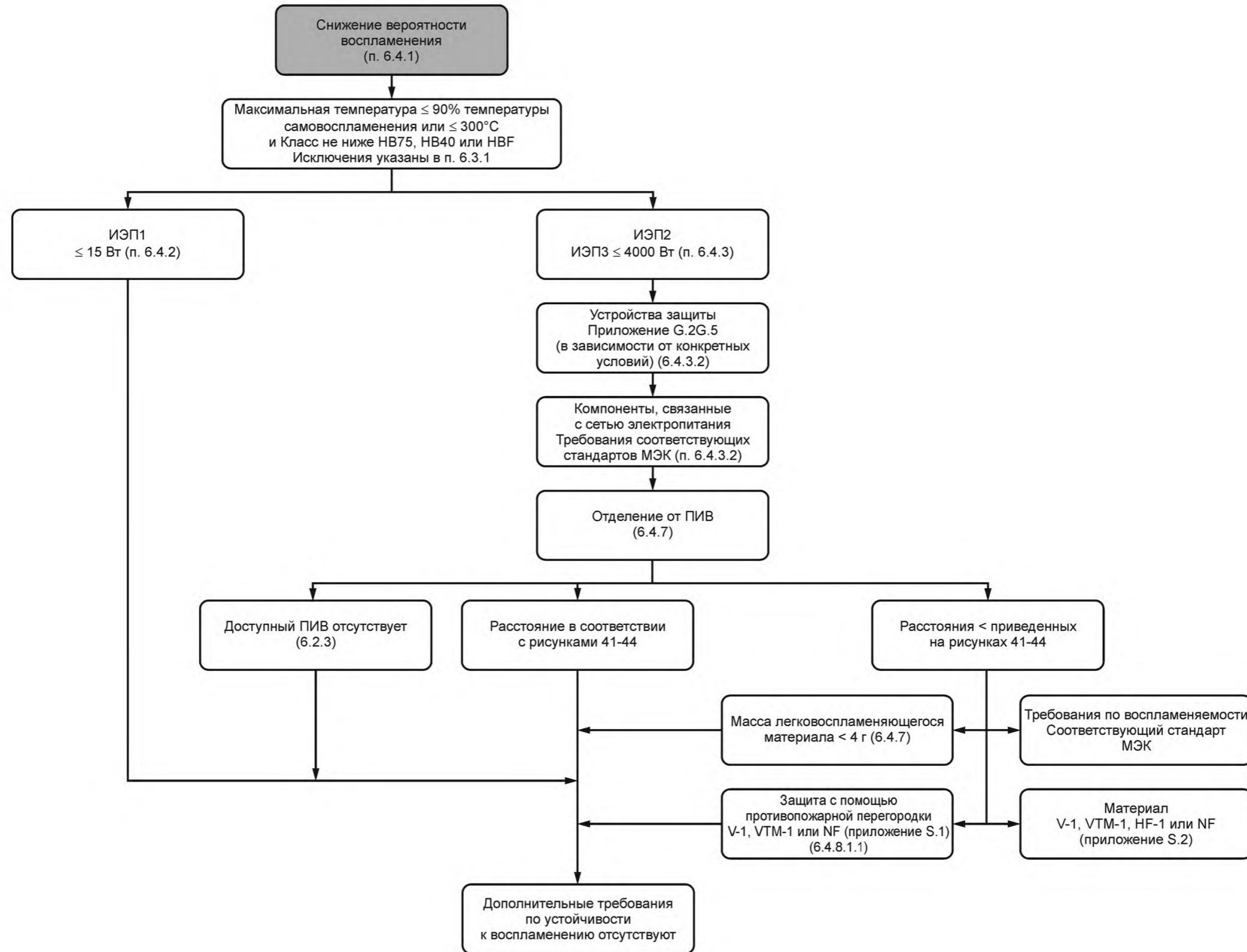
Рисунок 14 — Блок-схема метода, который заключается в предотвращении воспламенения
