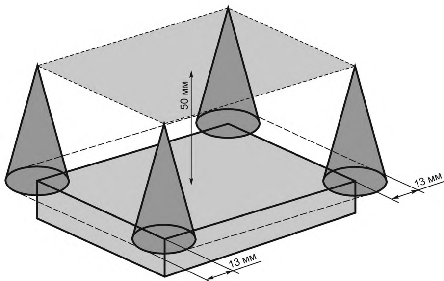
Рисунок 17 — Использование конуса пламени в случае крупного компонента
