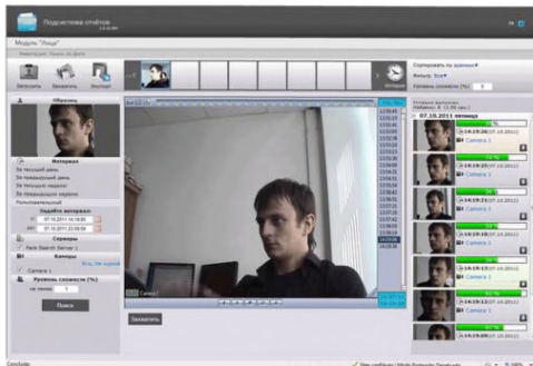
Рис. 76 - Модуль «Лица»
