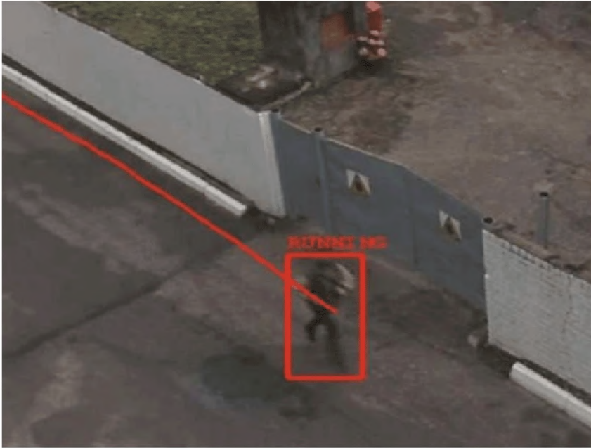
Рис. 24 - Детектор бега
