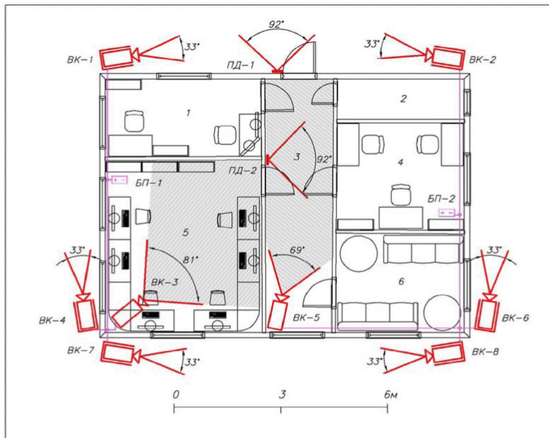
Рис. 16 - Система видеонаблюдения для ПЦО, вынесенного за пределы дислокации строевого подразделения отдела вневедомственной охраны с возможными зонами действия детектора дыма и пожара
