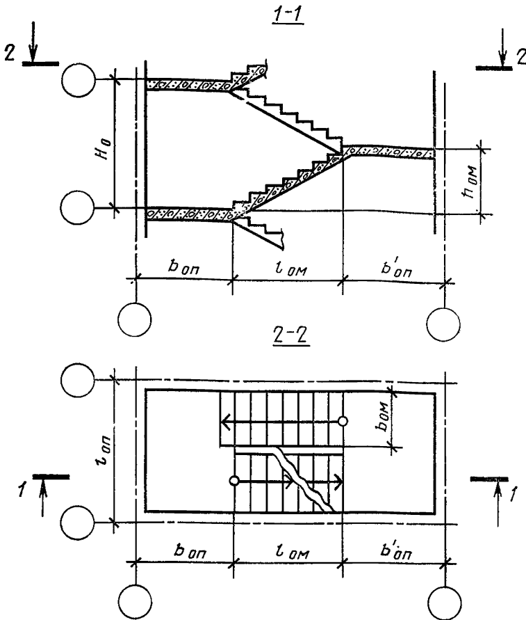
Схема лестницы
