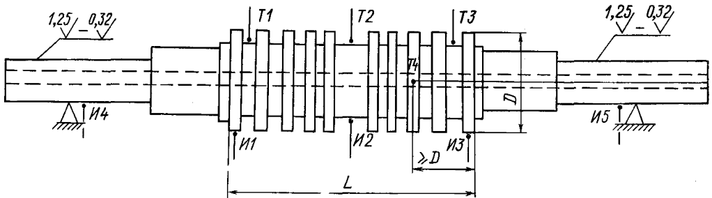
Схема расположения термопреобразователей и индикаторов бисения на объекте испытания
