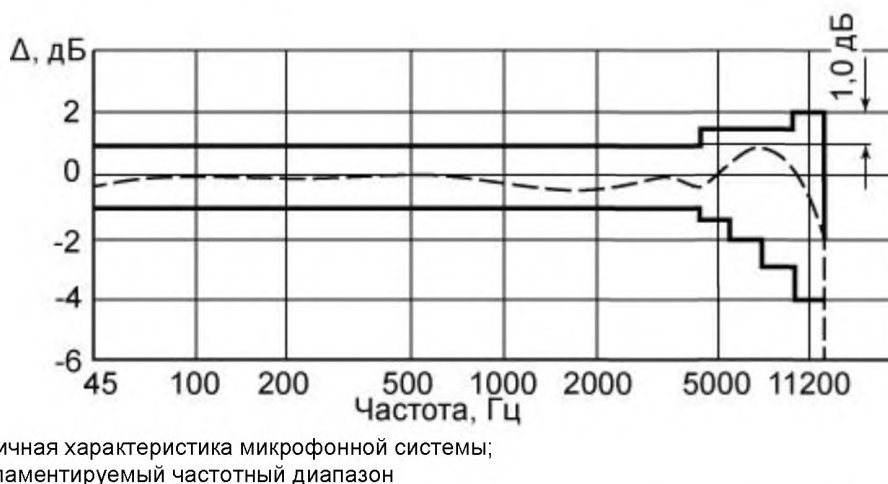
Рисунок Б.2 — Частотная характеристика микрофонной системы свободного поля
