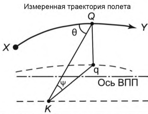
Рисунок 4 — Участки измеренной и исходной траекторий полета на оси ВПП
