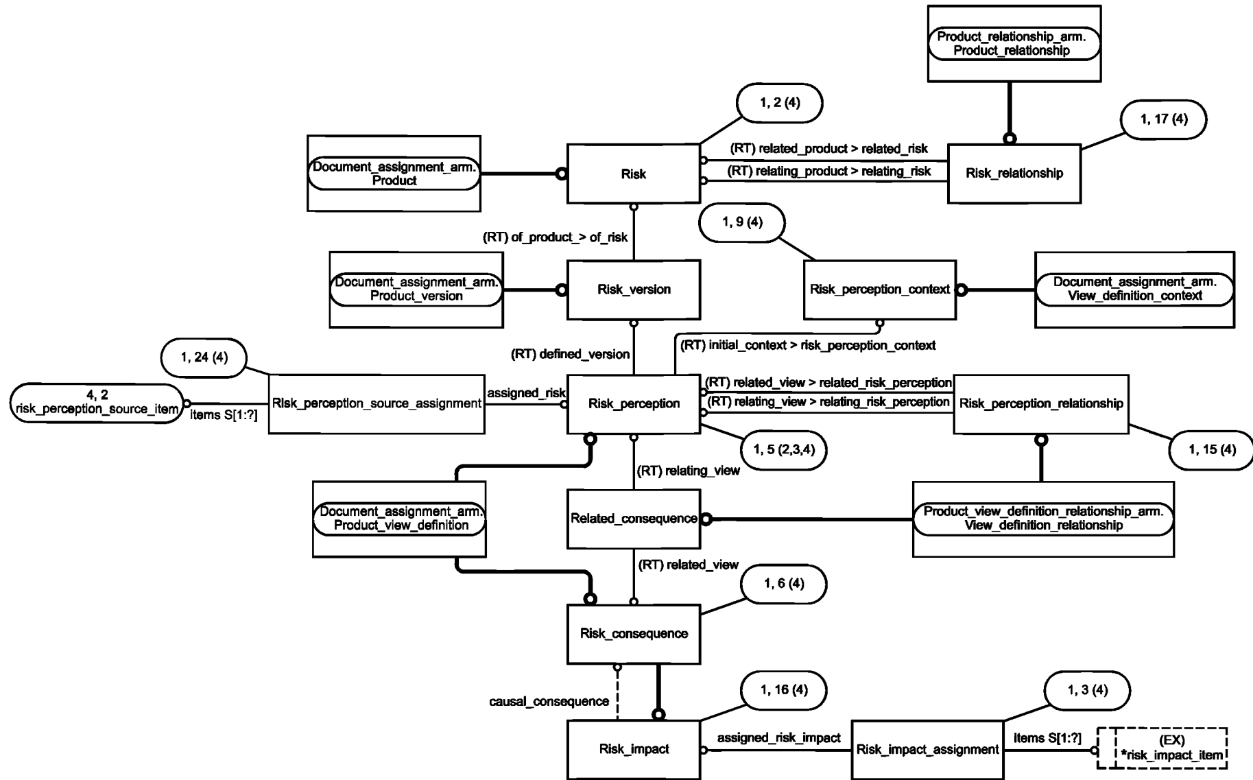
Рисунок С.2 — Представление ПЭМ на уровне объектов в формате EXPRESS-G (диаграмма 1 из 4)
