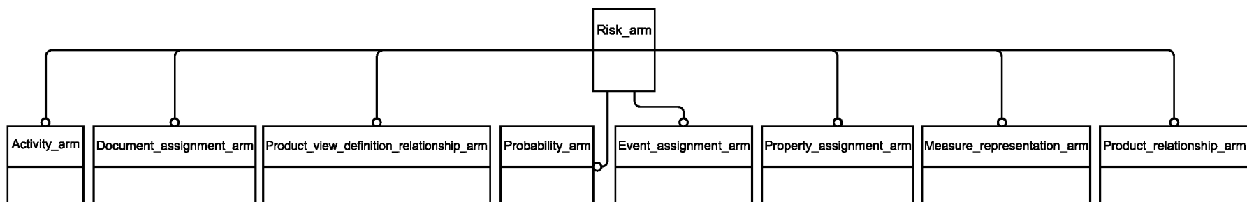
Рисунок С.1 — Представление ПЭМ на уровне схем в формате EXPRESS-G (диаграмма 1 из 1)
