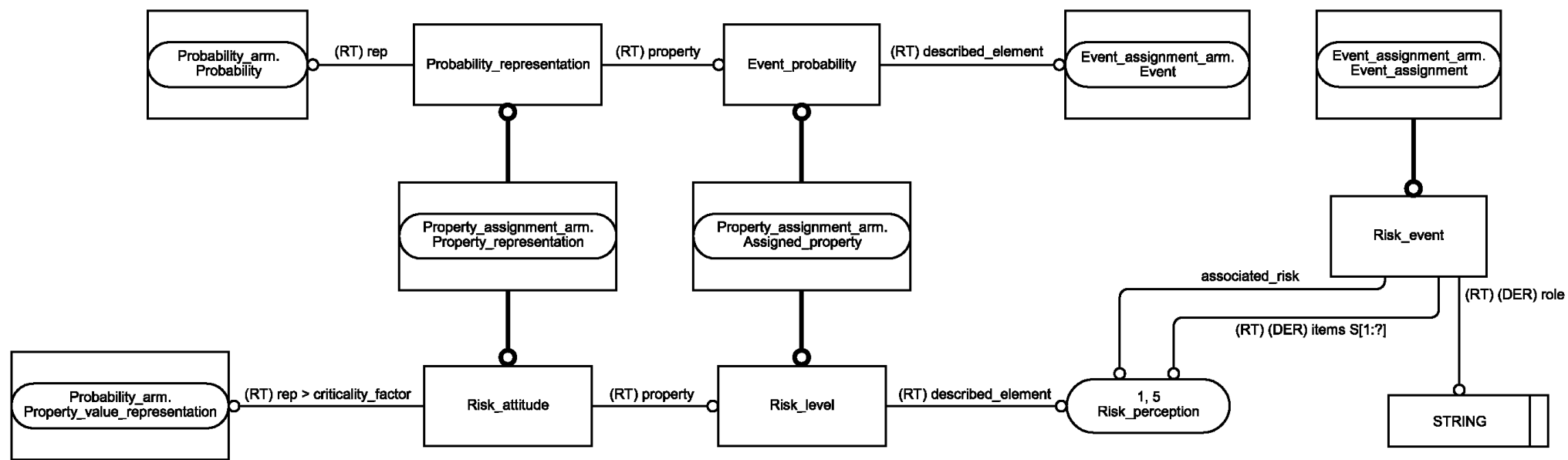
Рисунок С.4 — Представление ПЭМ на уровне объектов в формате EXPRESS-G (диаграмма 3 из 4)
