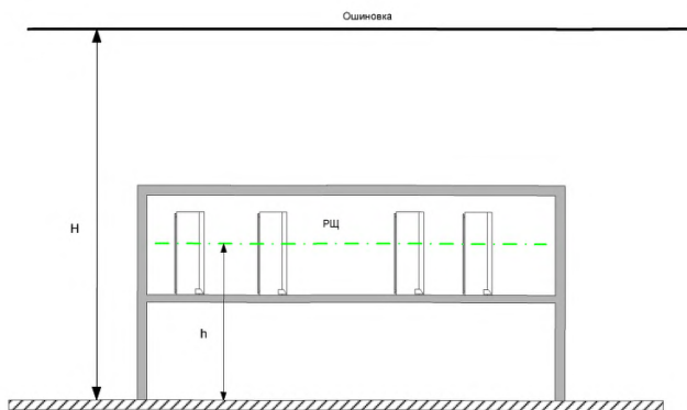
Рис.В.33 Расположение ошиновки над зданием РЩ
