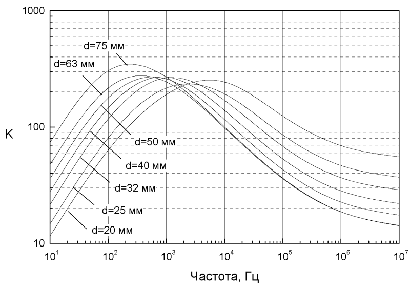
Рис.3.6 Коэффициенты экранирования стальных толстостенных труб различного диаметра
