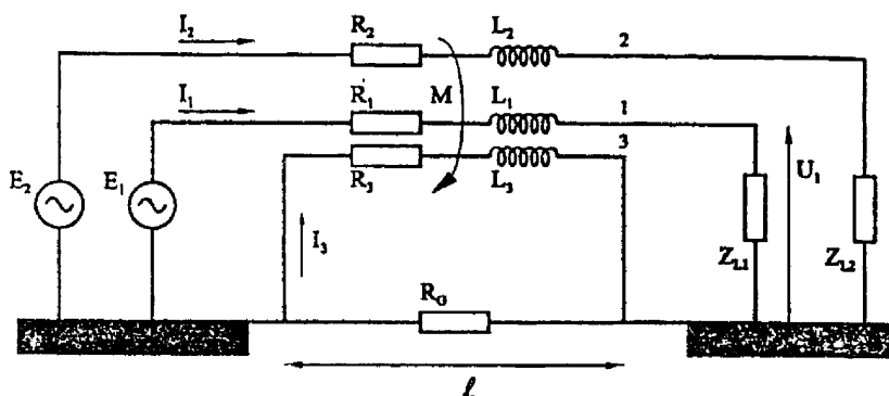
Рис. 3.2 Схема замещения для расчета коэффициента экранирования.
