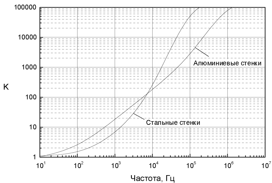
Рис.3.10 Коэффициенты экранирования металлических шкафов
