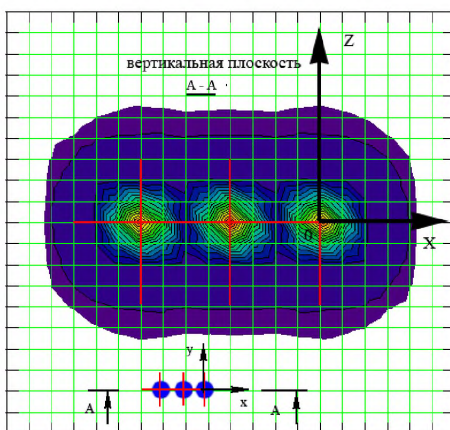
Рис.В.5 Характер распределения НМП в вертикальной плоскости
