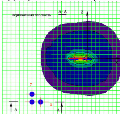
Рис.В.14 Характер распределения НМП в вертикальной плоскости
