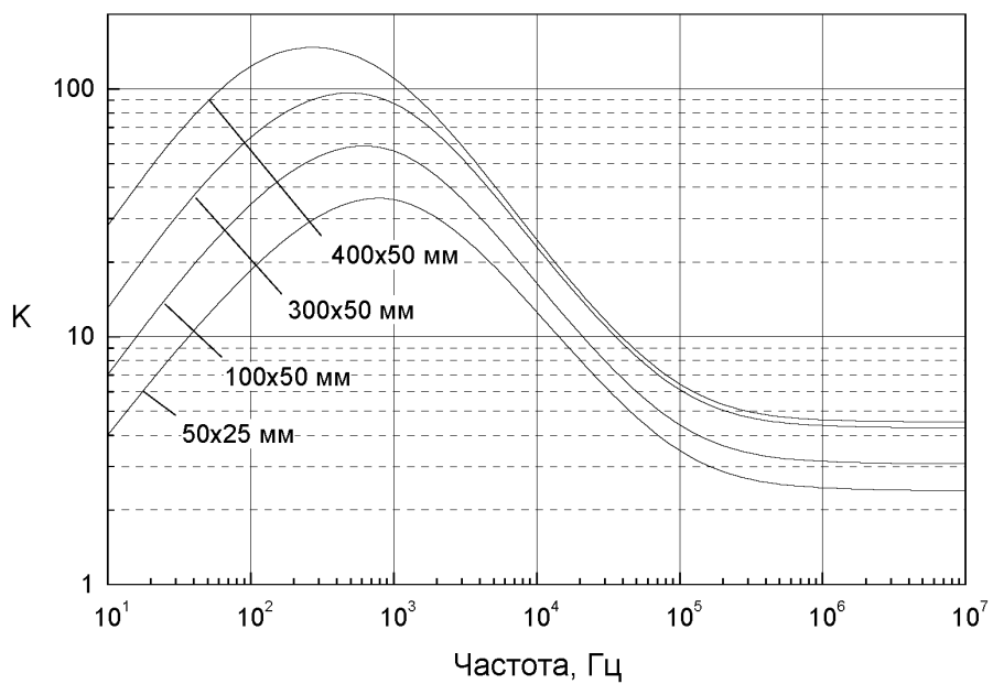
Рис.3.7 Коэффициенты экранирования стальных лотков различного сечения
