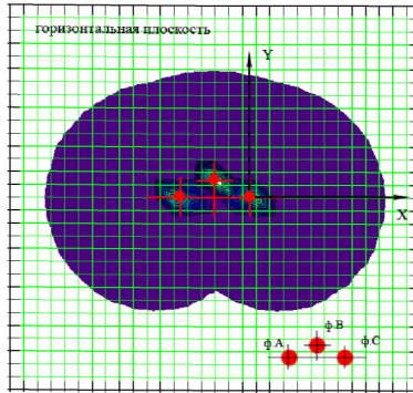
Рис.В.23 Характер распределения НМП в горизонтальной плоскости
