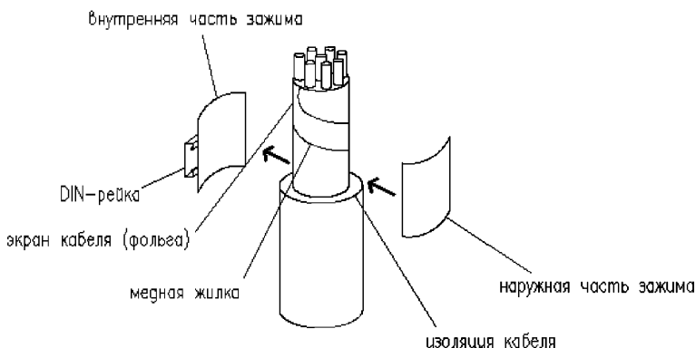
Рис.Е.4 Заземление экрана кабеля типа КВВГэ
