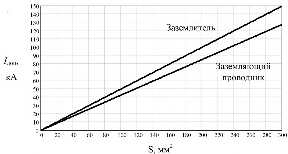
Рис. Ж.2 Допустимый ток КЗ для медных проводников горизонтального заземлителя и заземляющего проводника, подсоединенного к аппарату, при времени воздействия не более 0,1 с
