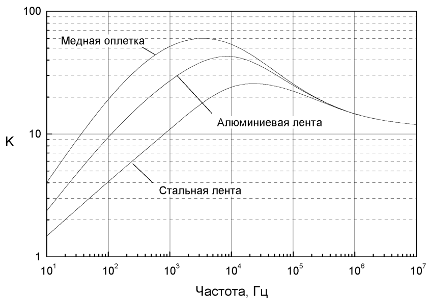
Рис. 3.4 Коэффициенты экранирования кабельных экранов
