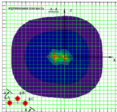
Рис.В.24 Характер распределения НМП в вертикальной плоскости
