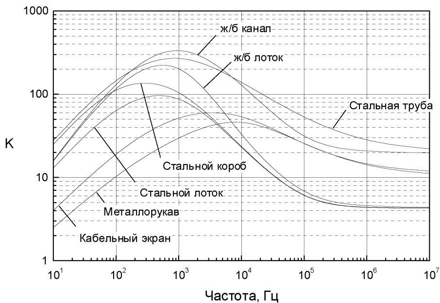
Рис. 3.3 Сравнительные коэффициенты экранирования различных экранирующих элементов
