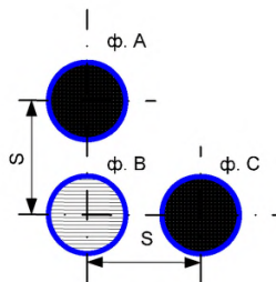
Рис.В.2 Расположение реакторов в вершинах равнобедренного прямоугольного треугольника
