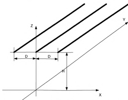
Рис.В.34 Расчетная модель
