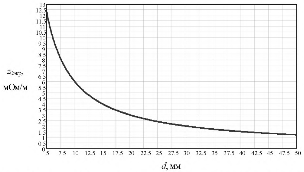
Рис. Ж.11 Зависимость погонного сопротивления алюминиевого экрана z_{0экp} от его наружного диаметра d
