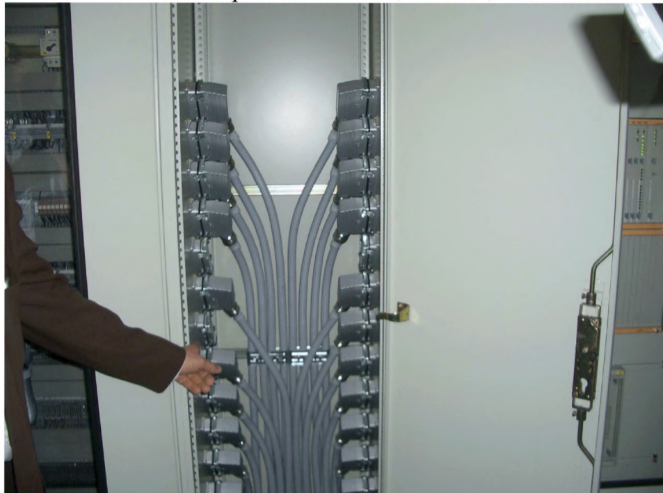
Рис.Е.2 Заземление экранов с помощью специальных зажимов
