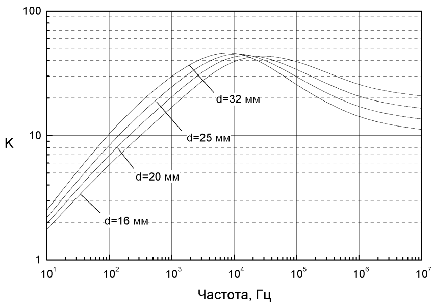
Рис. 3.5 Коэффициенты экранирования металлорукавов различного диаметра
