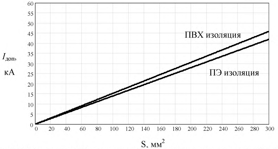
Рис. Ж.5 Допустимый ток КЗ для алюминиевой оболочки кабеля с поливинилхлоридной или резиновой изоляцией и полиэтиленовой изоляцией при времени воздействия не более 0,1 с
