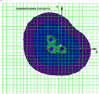
Рис.В.13 Характер распределения НМП в горизонтальной плоскости
