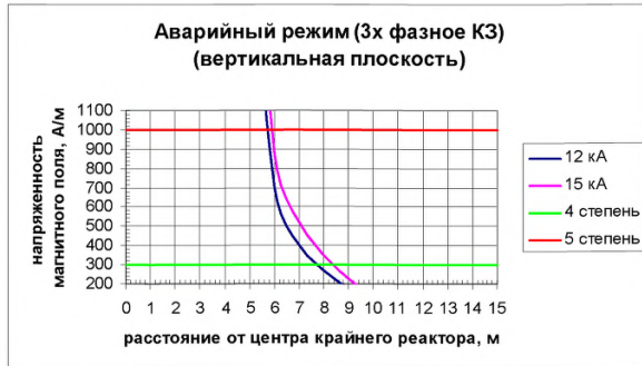
Рис. В.32 Распределение НМП при аварийных режимах в вертикальной плоскости при Z=0,96 Ом; n=45 ; R=0,9 м; S=2,4 м
