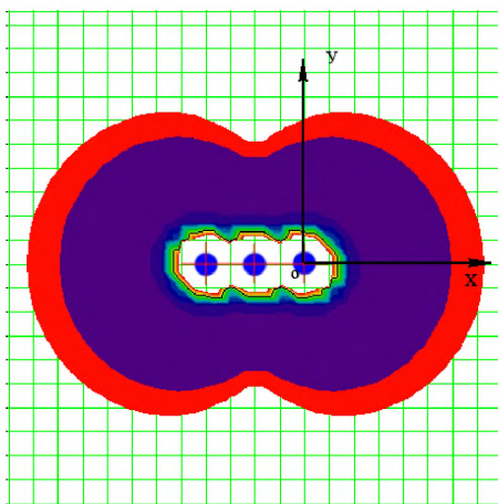
Рис.В.4 Характер распределения НМП в горизонтальной плоскости
