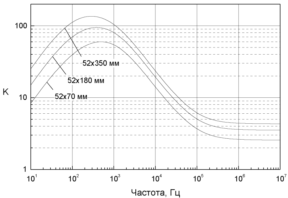
Рис. 3.8 Коэффициенты экранирования стальных коробов различного сечения
