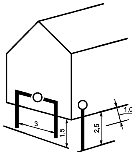
Рисунок 17b — Металлические штыревые заземляющие электроды а
