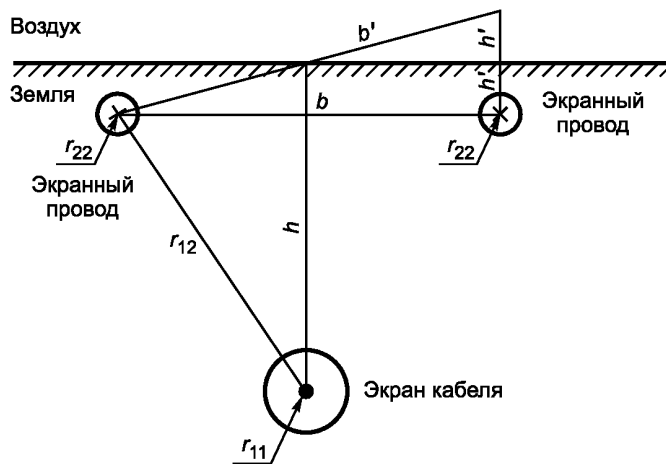
Рисунок В.2 — Принцип применения двух экранированных проводов
