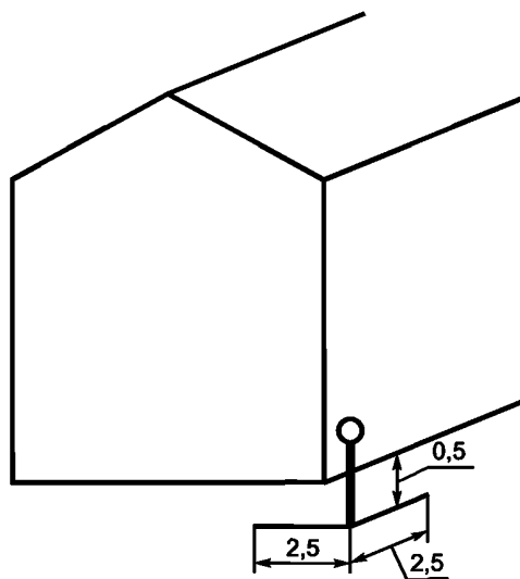
Рисунок 17с — Стальные полосы а
