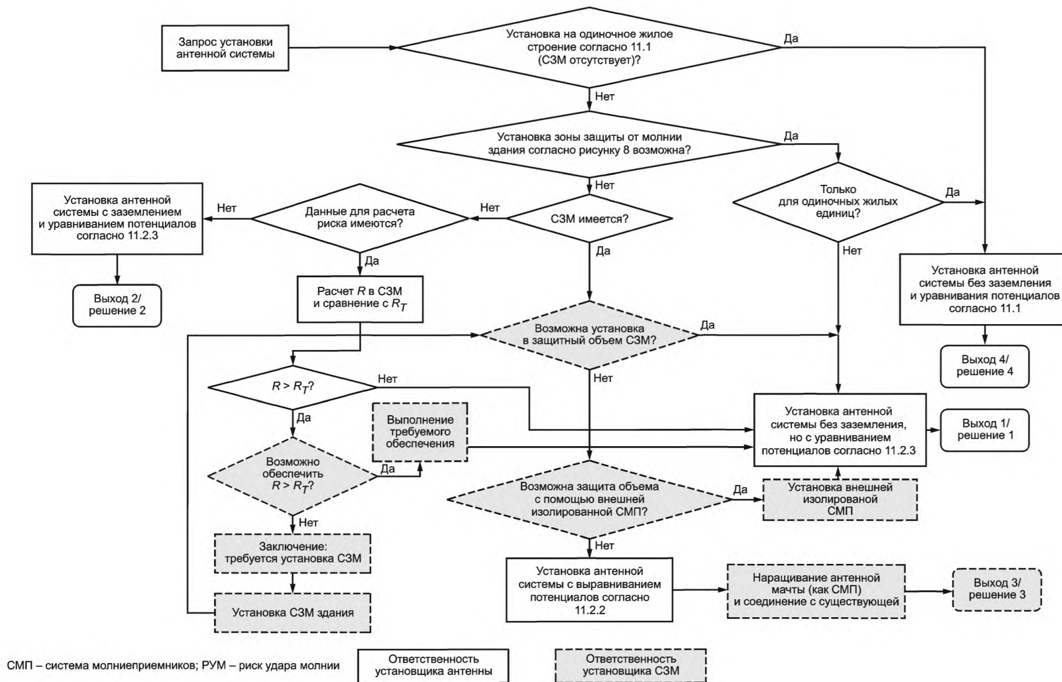
Рисунок 9 — Алгоритм выбора приемлемого метода защиты антенной системы от атмосферного электричества
