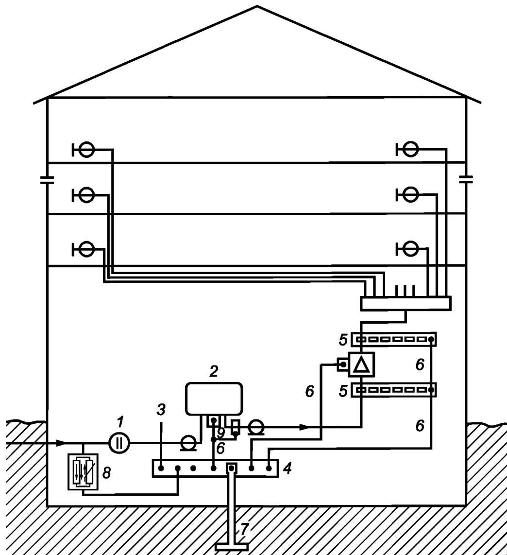
1 — гальванический изолятор; 2 — узел сопряжения; 3 — защитный проводник (PE), если необходим; 4 — заземляющий электрод; 5 — шина уравнивания потенциалов а ; 6 — защитный уравнивающий проводник [минимальное сечение согласно перечислению с) 6.2]; 7 — заземляющий электрод; 8 — устройство защиты от перенапряжения (минимальное сечение уравнивающего проводника, идущего к главной шине заземления 4, должно быть 16 мм 2 ; 9 — зажим заземления [см. перечисления ], к) 6.2]
