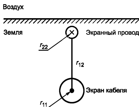
Рисунок В.1 — Принцип применения одного экранирующего провода
