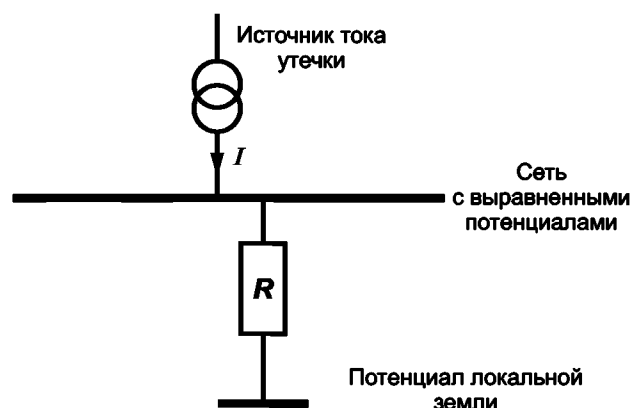
Рисунок А.1 — Сопротивление цепи заземления
