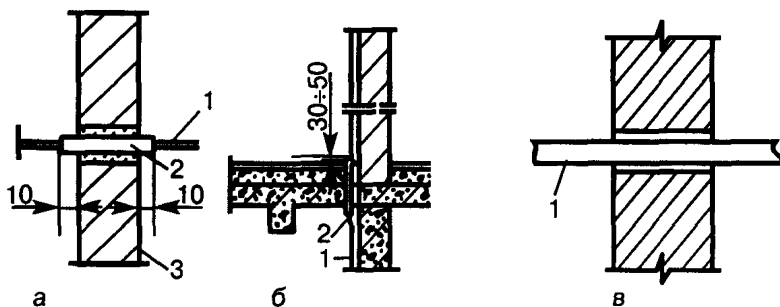
Рис. 13. Проходы заземляющего проводника сквозь стену (а), через перекрытие (б), в открытом проеме (в): 1 – заземляющий проводник из полосовой стали; 2 – гильза (стальная тонколистовая толщиной 1 мм); 3 – штукатурка
