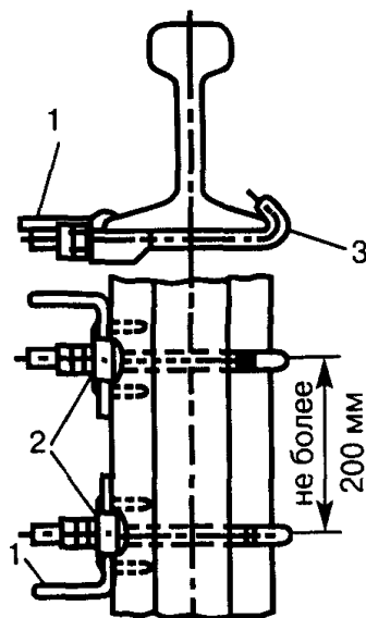
Рис. 3. Присоединение к тяговому рельсу проводников защитного заземления: 1 – провод заземления; 2 – зажим заземления; 3 – крюковой болт
