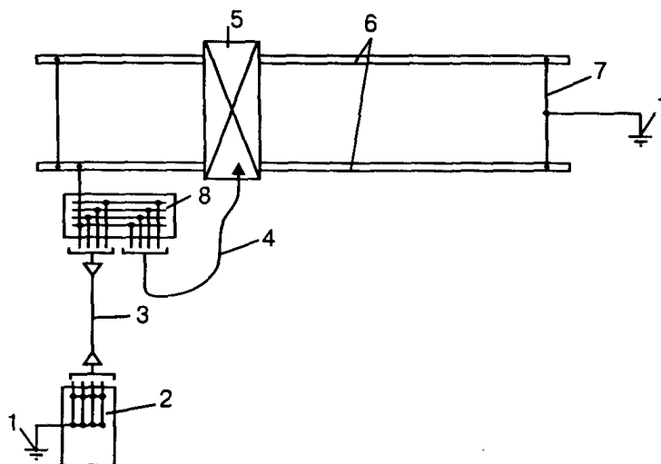
Рис. 18. Схема заземления крана, установленного на открытом воздухе и питающегося по гибкому кабелю: 1 – заземлитель; 2 – вторичная обмотка питающего трансформатора; 3 – неподвижный четырехжильный питающий кабель; 4 – гибкий переносной питающий кабель; 5 – кран; 6 – рельсовые пути крана; 7 – перемычка; 8 – вводно-распределительное устройство
