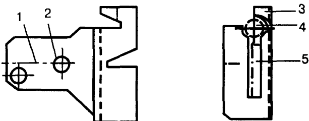
Рис. 12. Держатель шин заземления: 1 – место пристрелки; 2 – отверстие для крепления шурупами; 3 – отгибаемый элемент; 4 – место установки круглого проводника; 5 – место установки плоского проводника
