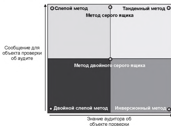
Рисунок 1 – Виды тестирования
