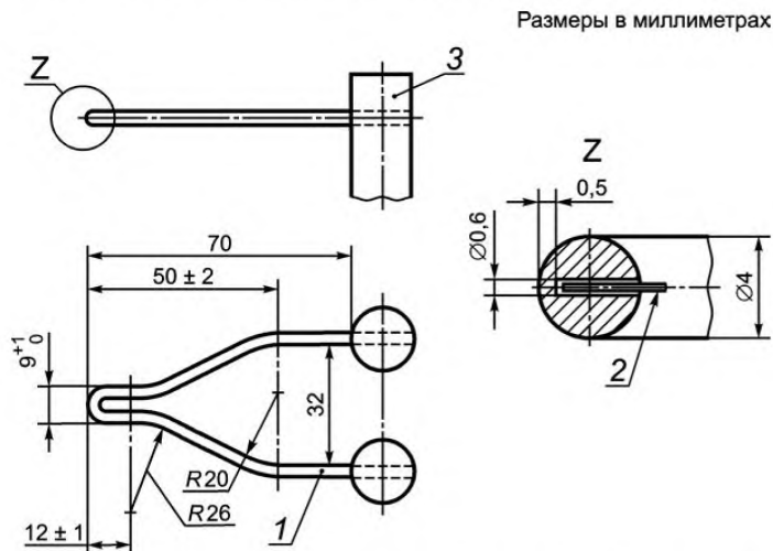
Рисунок 1 — Раскаленная проволока
