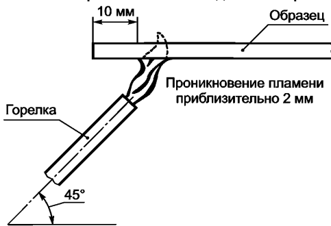
а) Горизонтальный образец. Приложение пламени к поверхности
