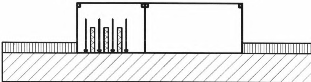
Рисунок АА.2 – Пример напольной установки шинпровода
