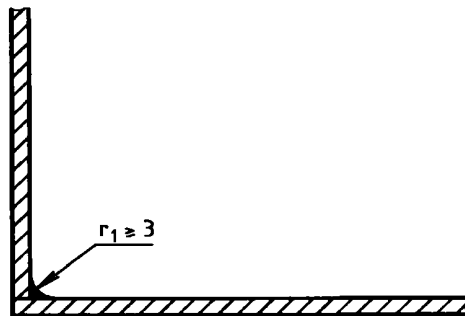
Рисунок А.1.2 – Пищевая зона
