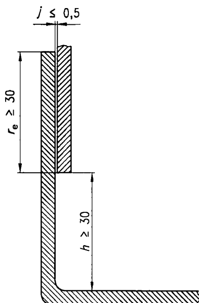
Рисунок А.5.3 – Зона распыления
