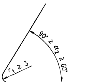
Рисунок А.2.2 – Зона распыления
