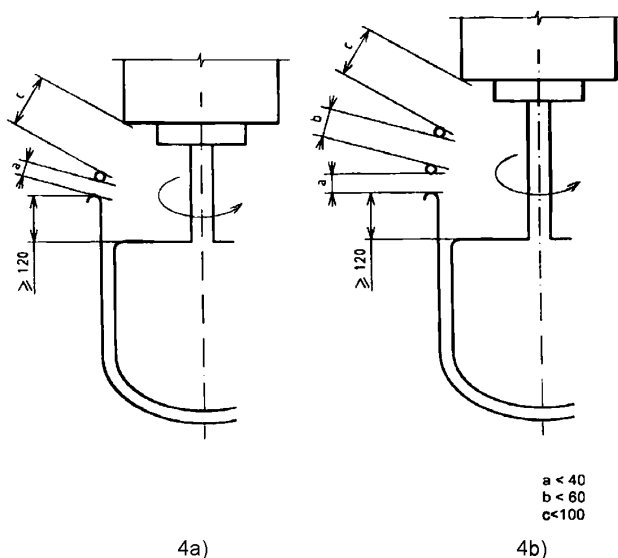
Рисунок 4 – Планетарные смесители класса 2 с предохранительными планками
