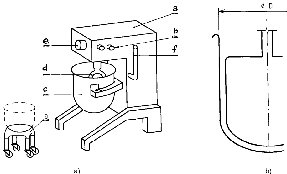
a – корпус привода лопасти(ей) мешалки; b – панель управления; c – дежа; d – лопасти мешалки; e – дополнительная приводная ступица; f – устройство для вертикального перемещения дежи или головки мешалки для удаления лопасти из дежи; g – технологическая тележка
