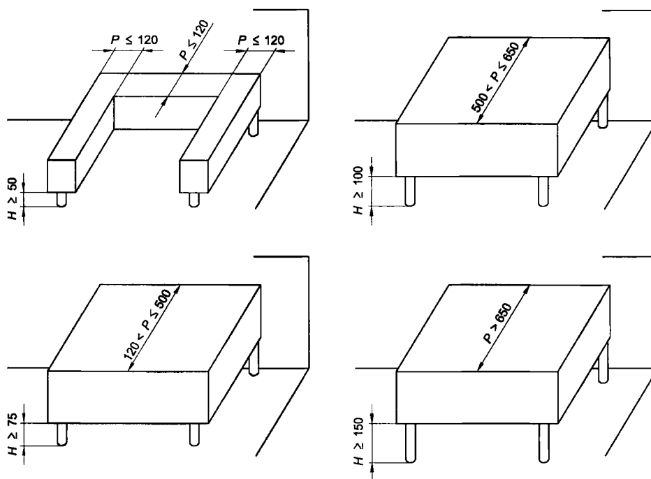
Рисунок А.8 – Подставки для смесителей
