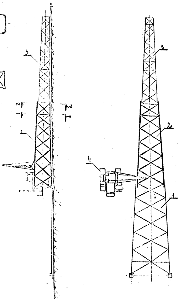
Рис. 19 Сборка 2.2 ой секции ствѣла опоры П220-2.
