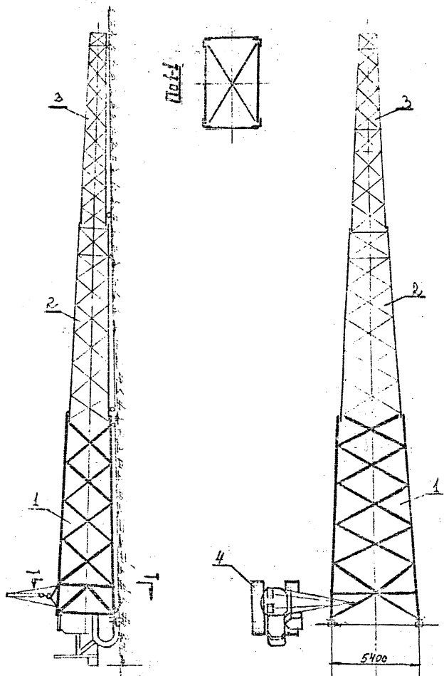
Рис. 20 Сборка 1 ой секции ствoла опоры П220-2.
