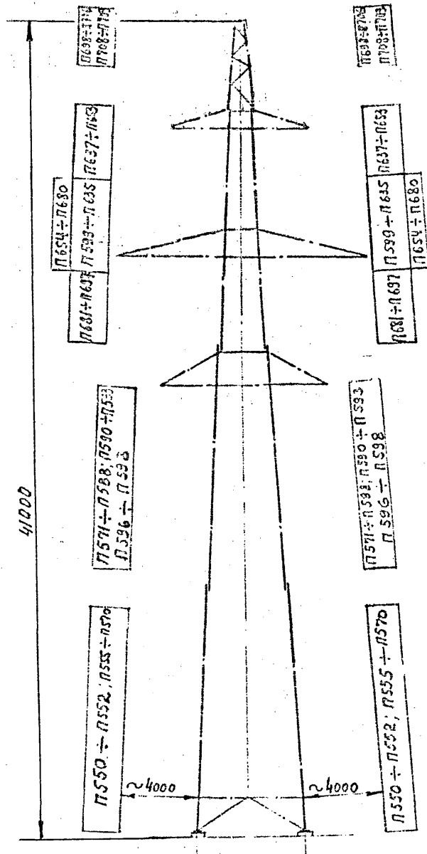
Рис.16 Раскладка пакетов с оттяжками стержня П220-2 на пакете.
