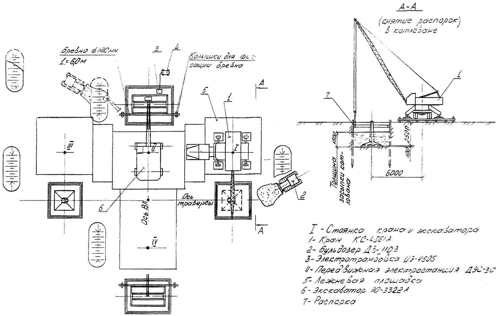
Рис. 5-2 Схема обратной засыпки котлована
