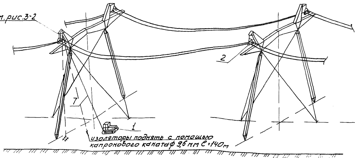
Рис. 3-1. Перекладка грозозащитных тросов
