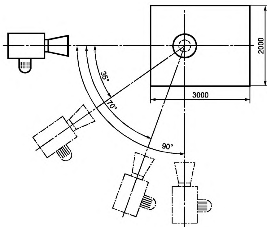
б) испытательный стенд для приборов типа С 3 , оборудованных вертикальным терминалом на наклонной крыше
