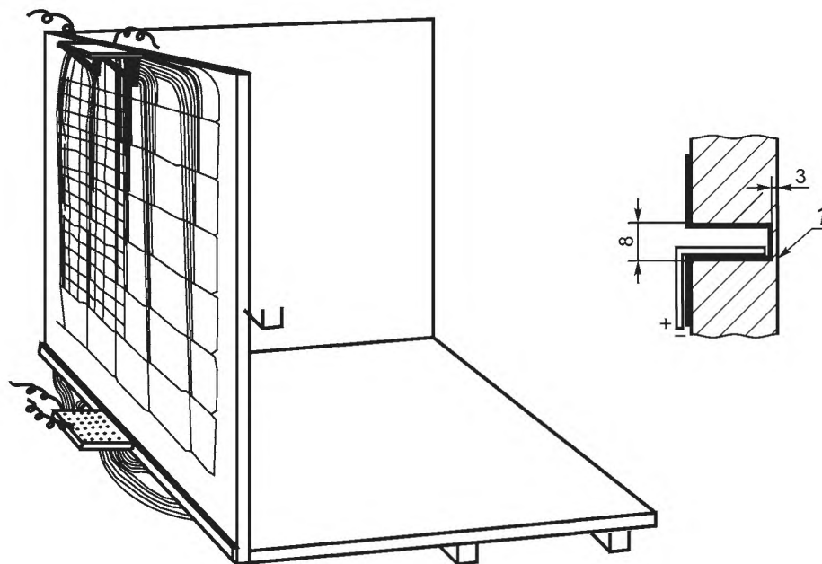
а) расположение термопар
