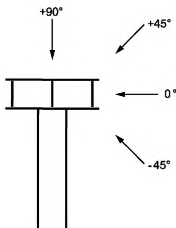
Рисунок С.3 — Скорости ветра
