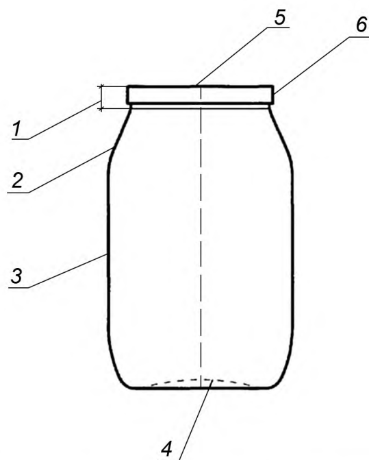
Рисунок А.2 — Конструкция банки
