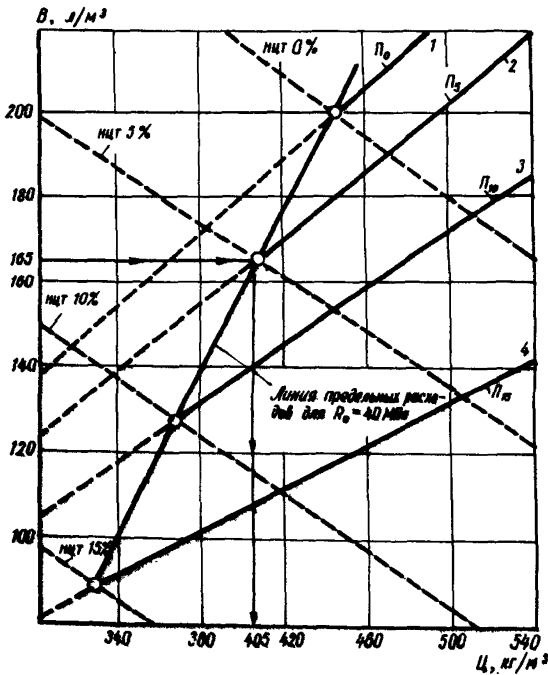
Рис.5. Выбор расхода цемента по расходу воды с учетом предельного содержания незаполненных гракулометрических пустот в песке (НЦТ)
