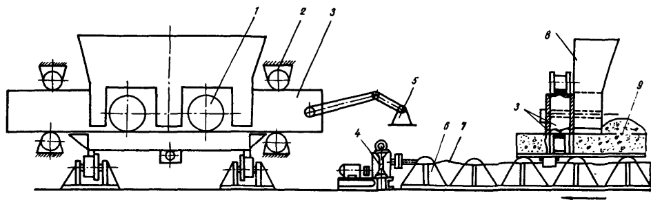
Рис.1. Конструктивная схема установки для роликового формования
