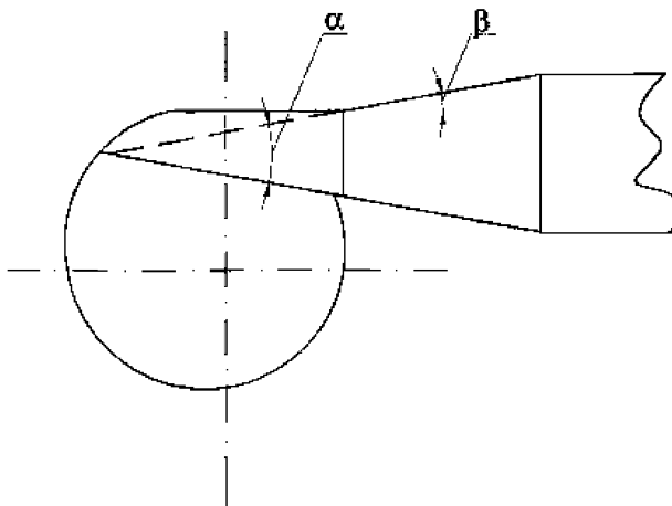
Рисунок 5.3 – Схема присоединения к вентилятору или дымососу нагнетательной части газоздухопровода
