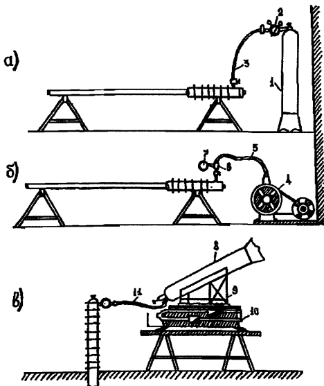
Рис.13. Схема пневматических испытаний (а), вакуумирования (б) и зарядки охлаждающих устройств теплоносителем (в):
