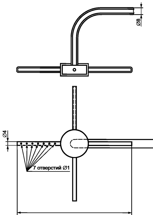
Рисунок 3 — Пробоотборник
