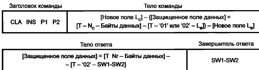
Рисунок 6 — Защищенная пара команда-ответ
