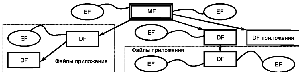
Рисунок 2 — Пример иерархии файлов DF
