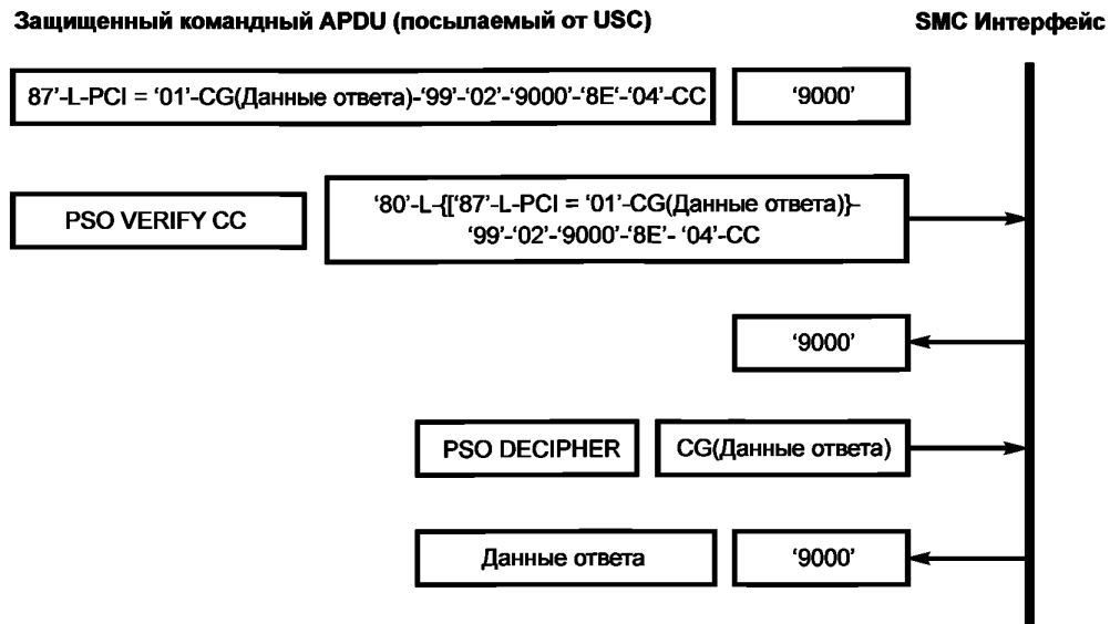
Рисунок В.2 — Создание защищенного ответного APDU
