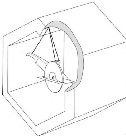
Рисунок 106 – Камера для испытания кожуха на прочность
