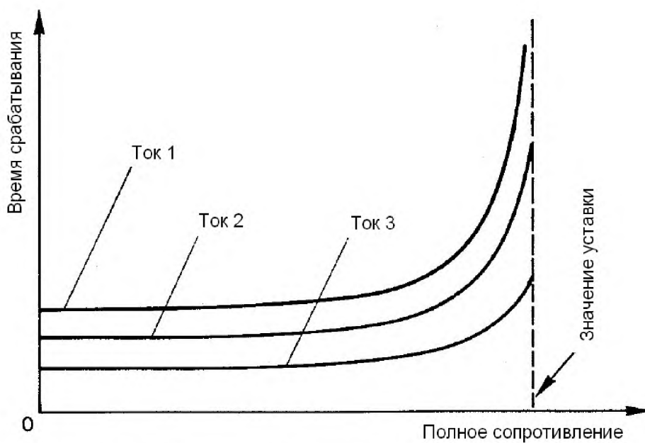
Рисунок 5 – Время срабатывания в нормальных условиях
