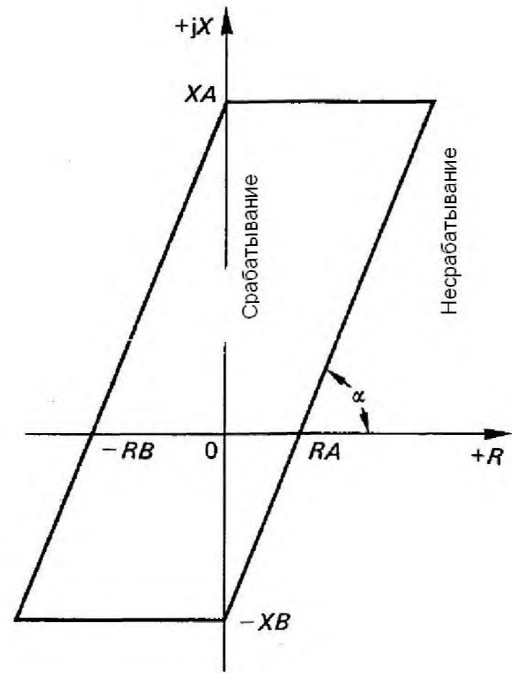
Уставки реле: RA, RB, XA, XB, \alpha
