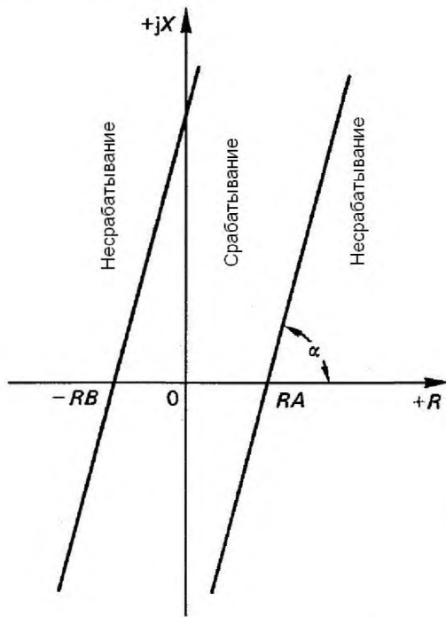
Уставки реле: RA, RB, \alpha
