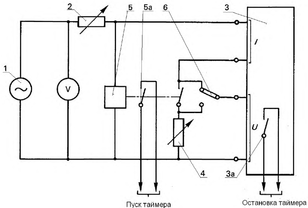
1 — стационарный источник напряжения; 2 — полное сопротивление регулируемого источника Z_S ; 3 — испытуемое реле; 3a — выходной контакт; 4 — регулируемое полное сопротивление Z_S , измеряемое посредством реле; 5 — управляющее устройство точечного переключения; 5a — выключатель мгновенной подачи входных воздействующих величин; 6 — переключающий элемент
