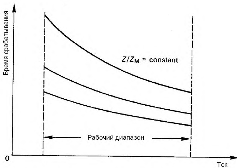
Рисунок 5 – Время срабатывания в нормальных условиях
