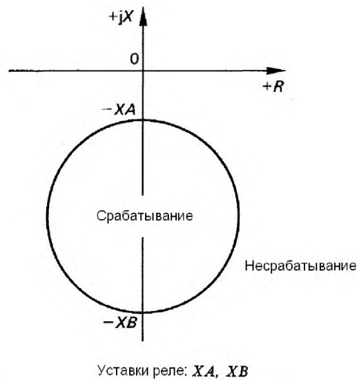
Рисунок 1f — Круговая смещенная характеристика
