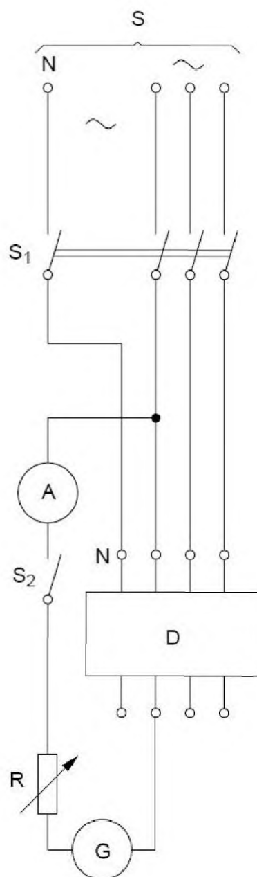
S — источник питания; S 1 — испытательный выключатель, коммутирующий все полюса; S 2 — испытательный однополюсный выключатель; D — испытуемое УЗО; G — произвольный генератор сигнала (генерирующий 10 Гц, 50 Гц и 1 кГц); A — амперметр; R — резистор 10 Ом (или любое близкое значение)
