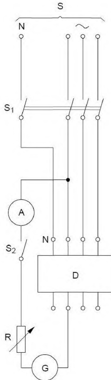
S — источник питания; S 1 — испытательный выключатель, коммутирующий все полюса; S 2 — испытательный однополюсный выключатель; D — испытуемое УЗО; G — импульсный генератор полуволны (генерирующий 50 Гц или 60 Гц); A — амперметр; R — резистор 10 Ом (или любое близкое значение)
