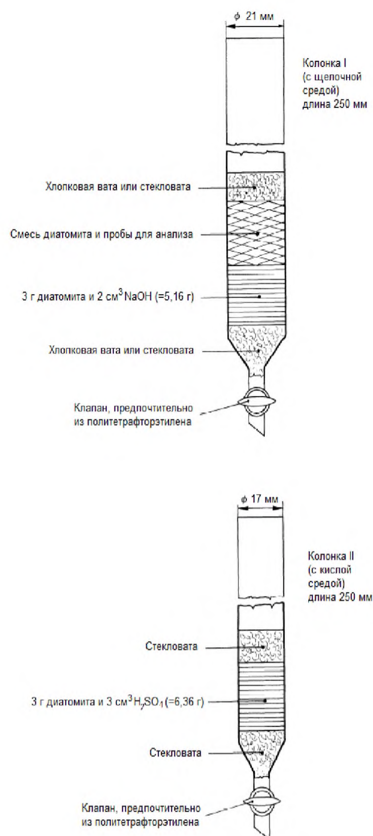
Рисунок 1 – Хроматографические колонки
