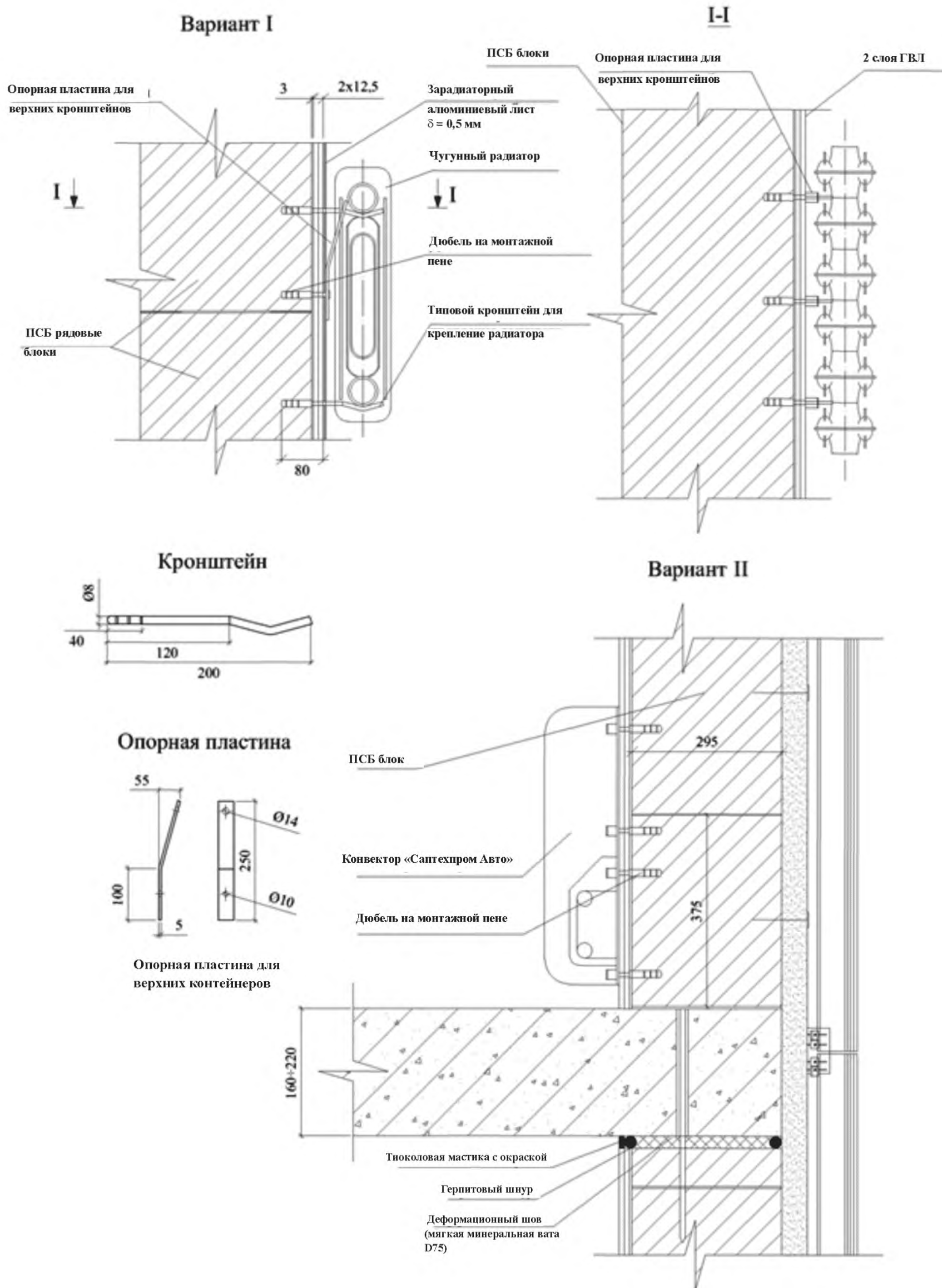
Рисунок 6.21 – Крепление отопительного оборудования
