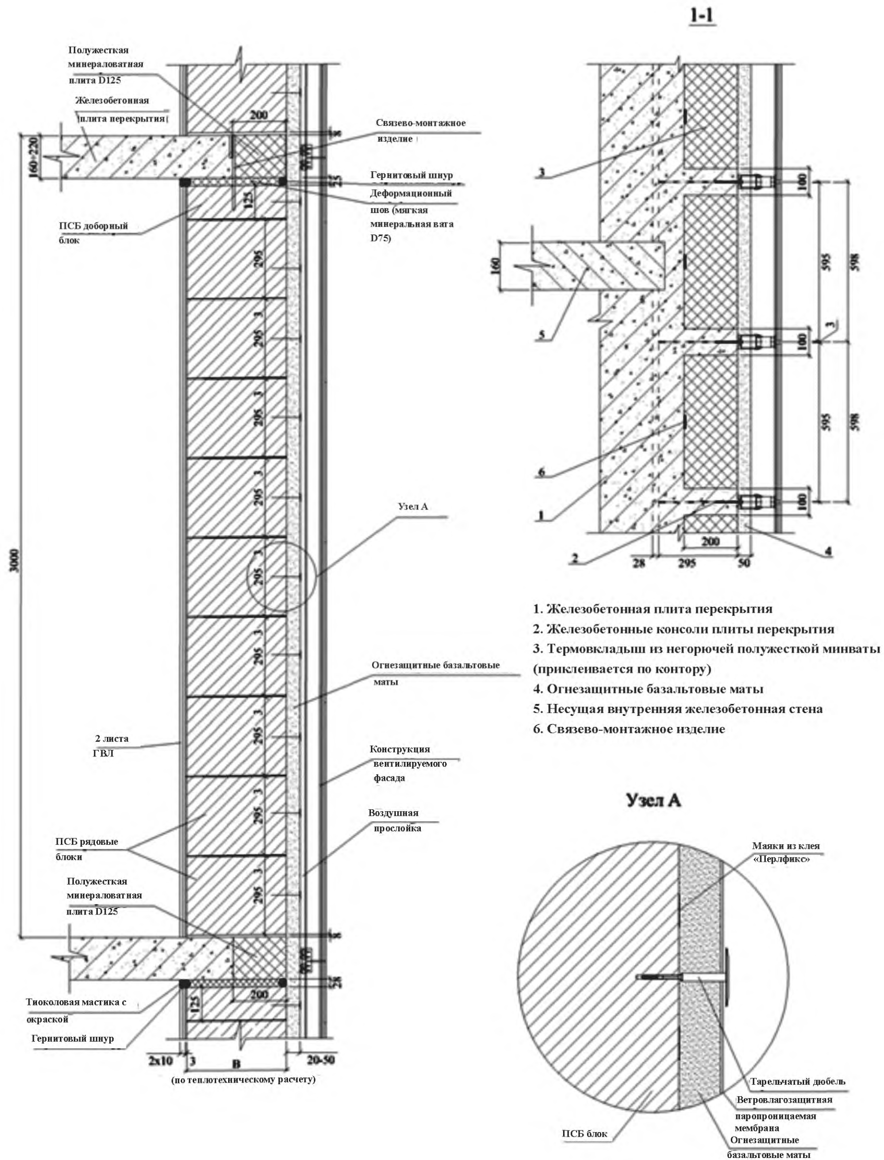
Рисунок 6.8, лист 2 – Ненесущая стена из ПСБ блоков с вентилируемым фасадом.
