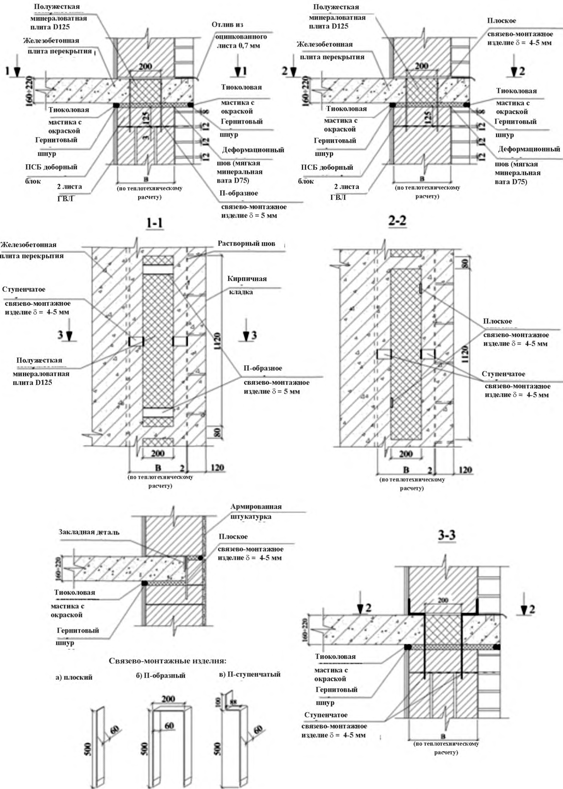
Рисунок 6.18 – Крепление кладки из ПСУБ блоков к железобетонным перекрытиям
