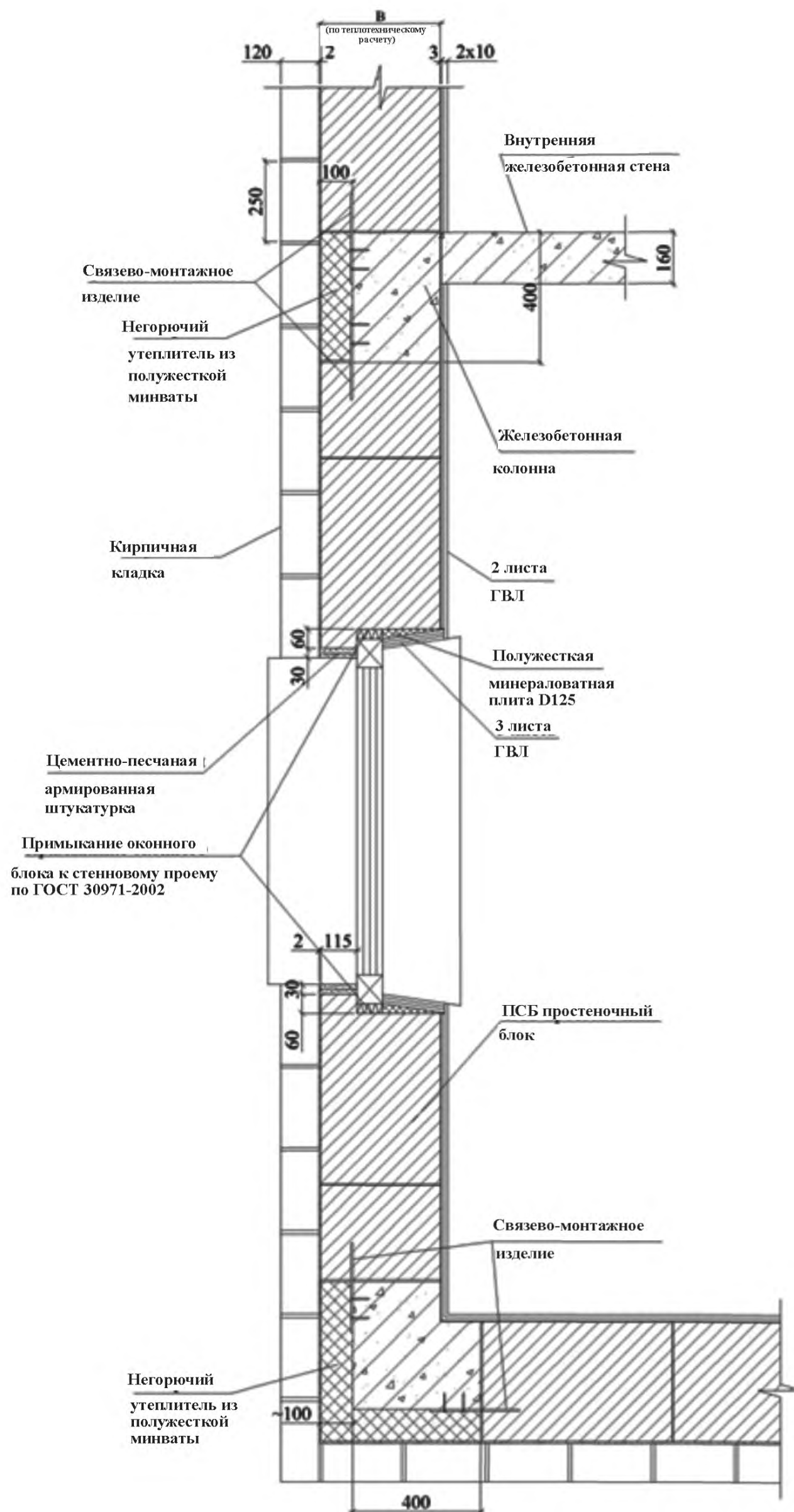
Рисунок 6.5 – Несущая стена из ПСБ блоков для зданий с несущими железобетонными колоннами и кирпичной облицовкой фасада. Горизонтальный разрез
