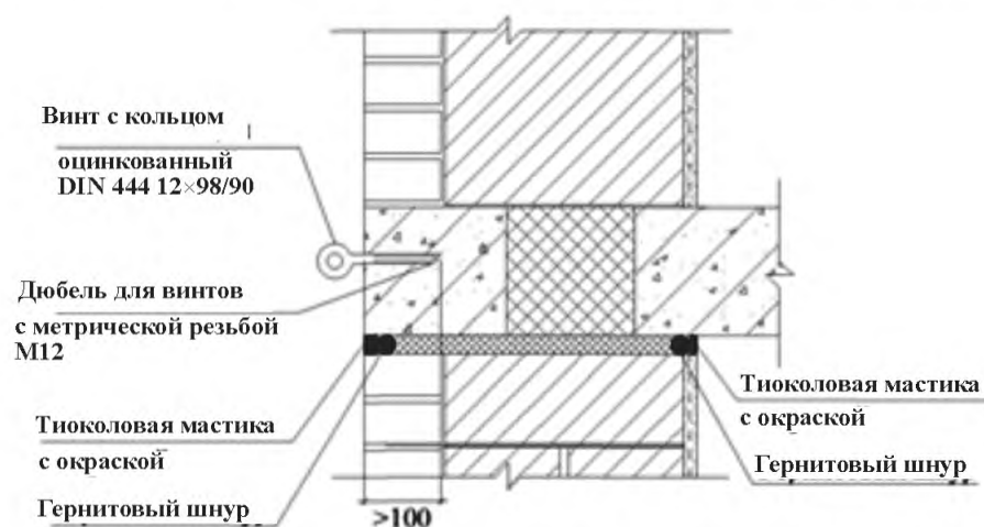
Рисунок 6.22 – Крепление навесных устройств к фасадам стен
