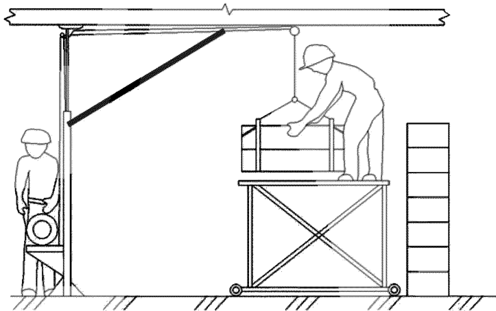
Рисунок 7.2 – Подача блоков на подмости краном-укосиной
