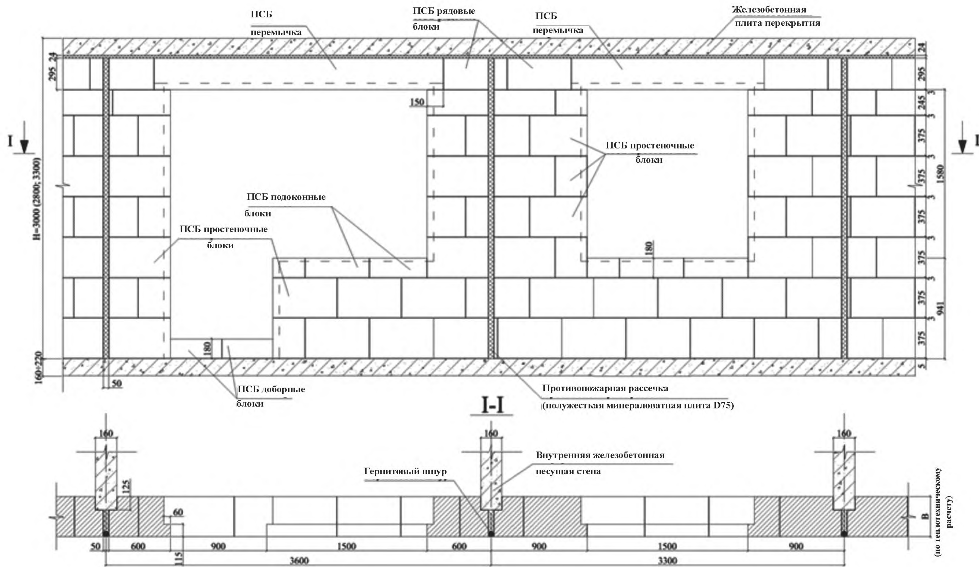
Рисунок 6.2 – Раскладка полистиролбетонных блоков высотой 375 мм и перемычек при монтаже наружной стены здания с внутренними поперечными несущими стенами
