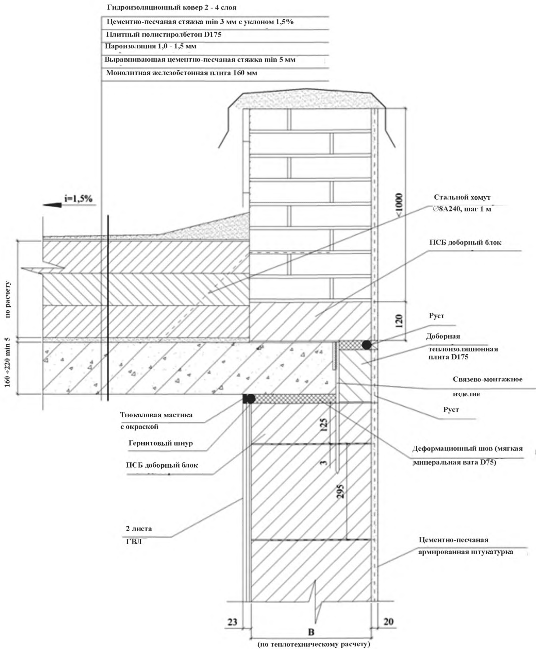
Рисунок 6.12 – Утепление покрытия здания с использованием плитного полистиролбетона
