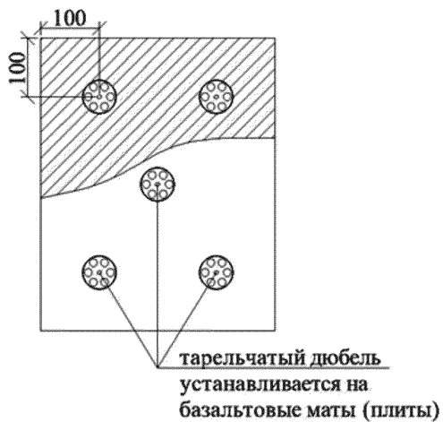
Рисунок 7.3 – Монтаж утеплителя и установка тарельчатых дюбелей
