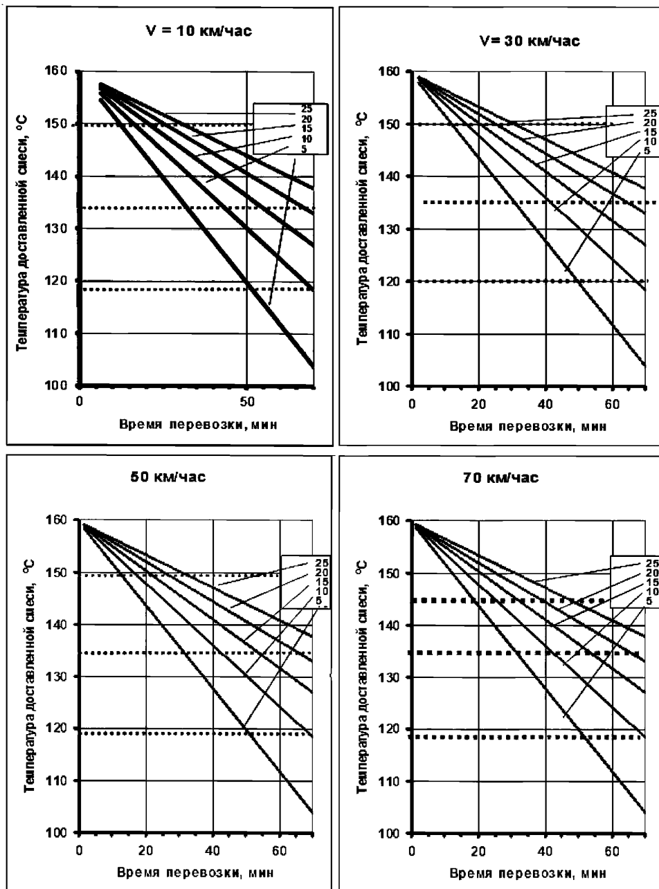
Рисунок П.1 – Время перевозки горячей асфальтобетонной смеси в автомобилях-самосвалах при температуре отгрузки t_{нач} = 160 °C (цифры на лучах – температура воздуха)
