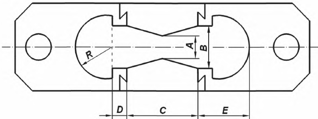
A - (10,0 \pm 0,2) мм; B - (20,0 \pm 0,2) мм; C - (30,0 \pm 0,3) мм; D - (7,3 \pm 0,5) мм; E = R + D - (22,8 \pm 0,9) мм; R - (15,5 \pm 0,7) мм; толщина – (10,0 \pm 0,1) мм Рисунок 1 – Тип формы для литья (размеры обязательные, форма произвольная)
