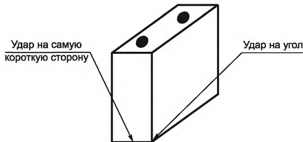
Рисунок 9 — Места на образце для удара
