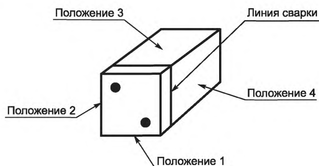
Рисунок 4 — Положение аккумулятора или моноблочной батареи при испытании
