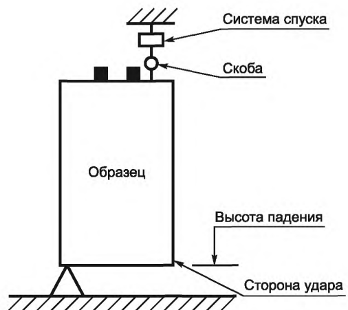
Рисунок 9 — Места на образце для удара
