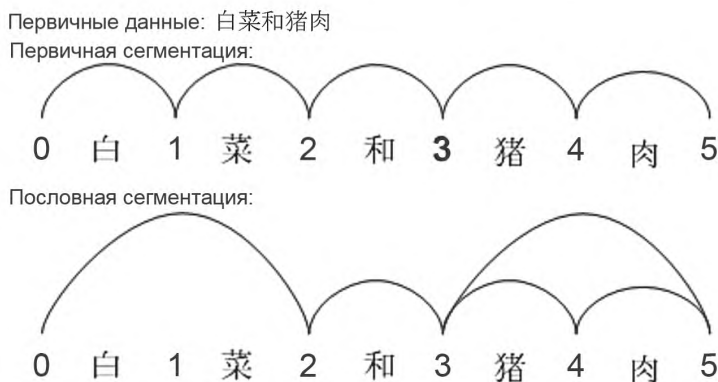
Рисунок 6 — Иллюстрация первичной сегментации и пословной сегментации
