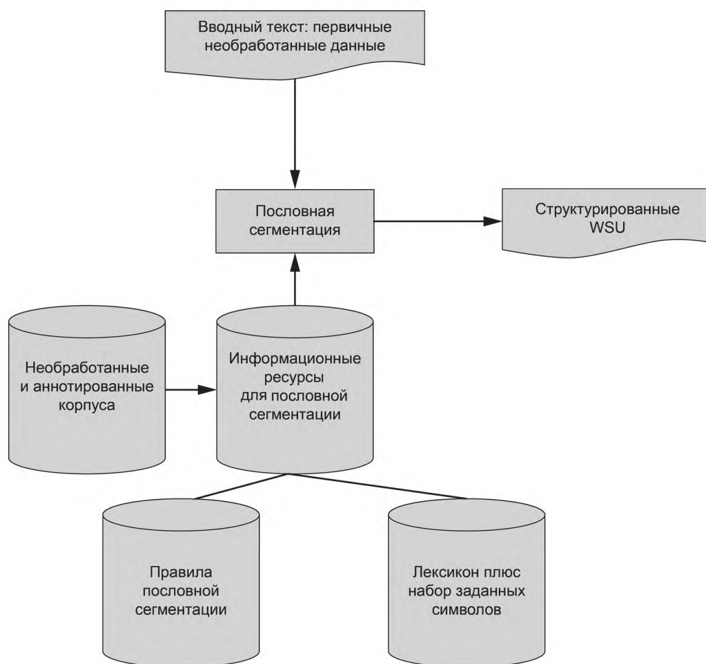
Рисунок 5 — Процесс пословной сегментации
