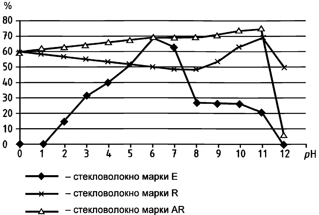
Рисунок А.1 – Коррозионная стойкость стекловолокна различных марок
