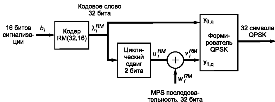
Рисунок 20 — Устойчивый (робастный) заголовок FECFrame
