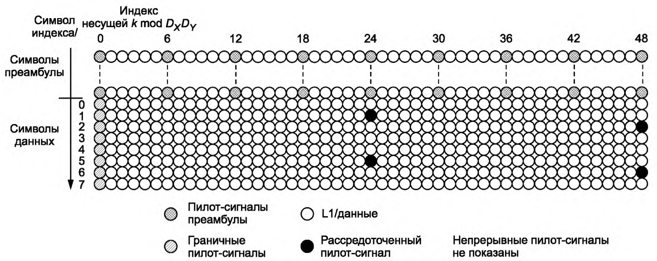
Рисунок Е.5 — Рассредоточенный пилот-сигнал для GI 1/128 с низкочастотной границей k \bmod D_x D_y = 0
