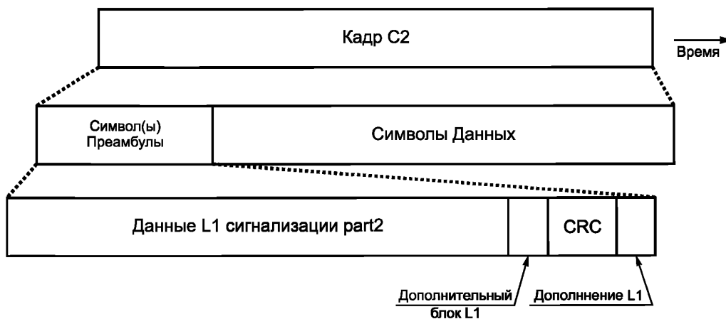
Рисунок 22 — Структура данных сигнализации L1-part2
