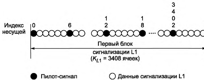
Рисунок 37 — Блок сигнализации L1
