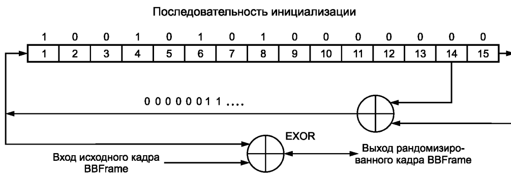
Рисунок 13 — Структурная схема возможной реализации кодера псевдослучайной последовательности
