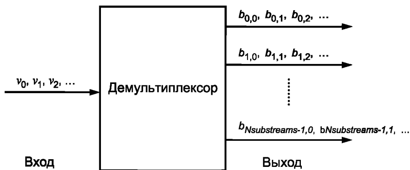
Рисунок 16 — Демультимплексирование битов в субпотoki
