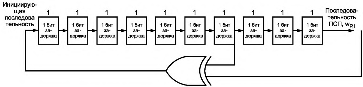
Рисунок 35 — Схема генератора ПСП для модуляции пилот-сигналов
