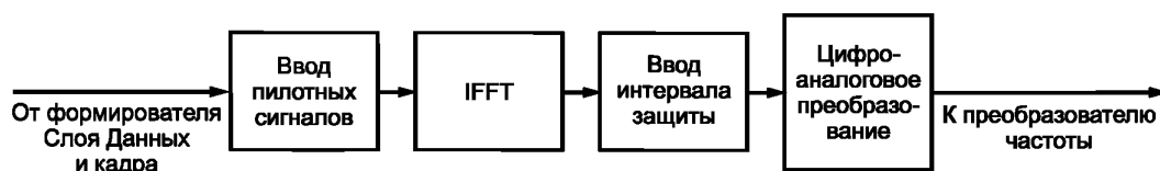
Рисунок 5 — Блок-схема подсистемы формирования сигнала OFDM
