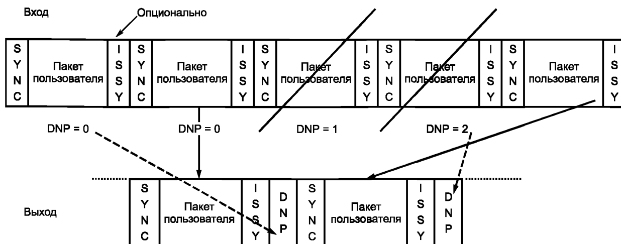
Рисунок 6 — Схема удаления нулевых пакетов
