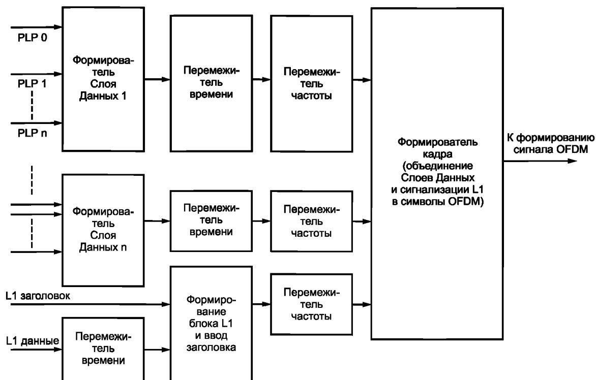
Рисунок 4 — Блок-схема подсистемы формирования Слоя данных и ядра
