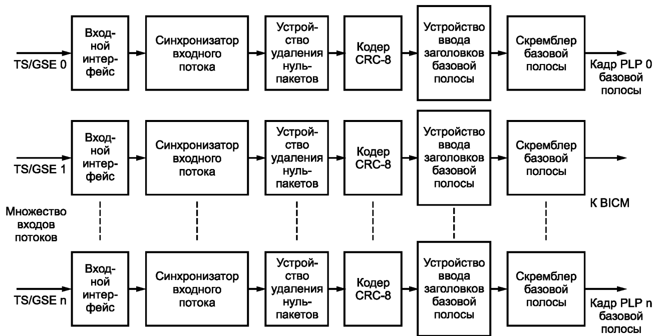
Рисунок 2 — Блок-схема подсистемы адаптации множества входных потоков
