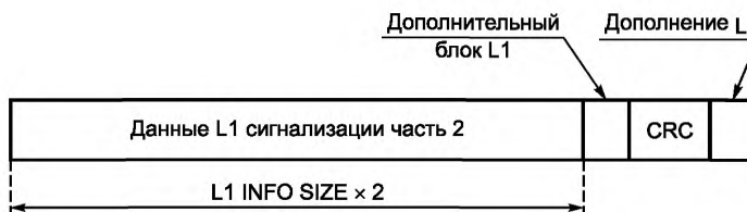
Рисунок 24 — Размер поля L1_INFO_SIZE
