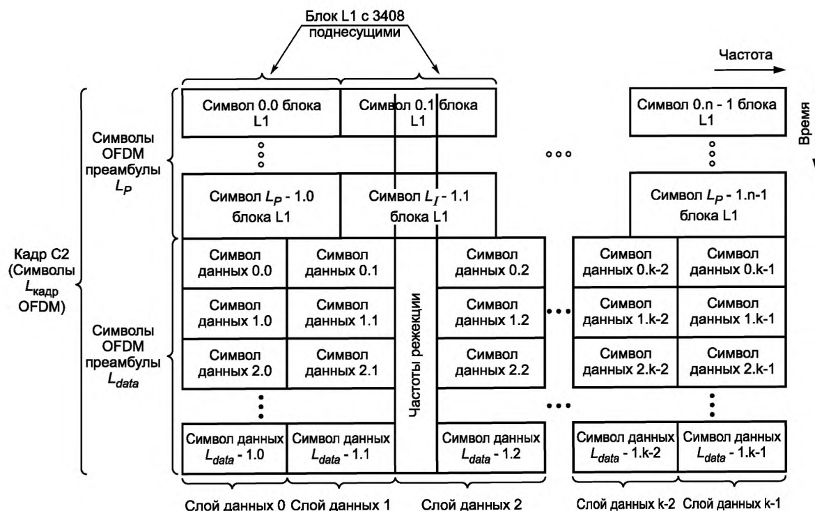
Рисунок 33 — Структура кадра C2
