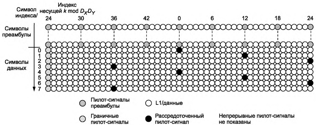
Рисунок Е.3 — Рассредоточенный пилот-сигнал для GI 1/64 с низкочастотной границей k \bmod D_x D_y = 24
