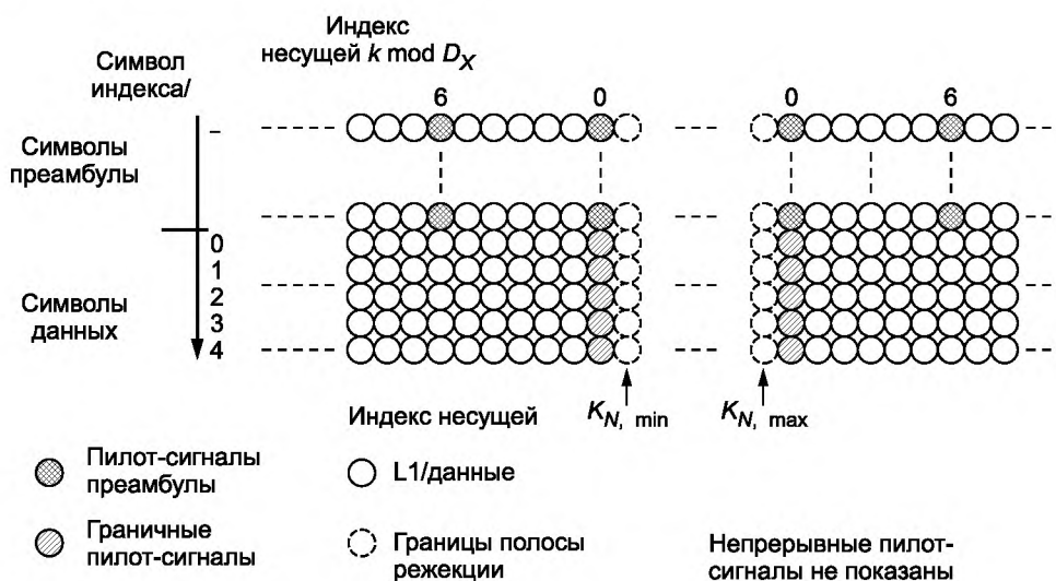
Рисунок 42 — Расположение граничных пилот-сигналов на границах полосы режекции
