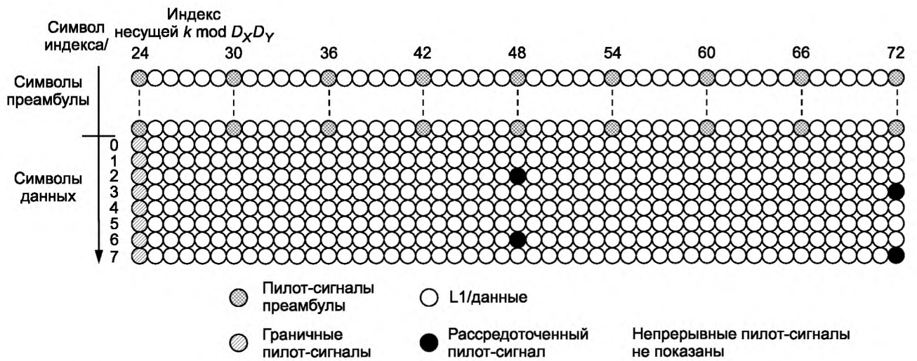
Рисунок Е.6 — Рассредоточенный пилот-сигнал для GI 1/128 с низкочастотной границей k \bmod D_x D_y = 24
