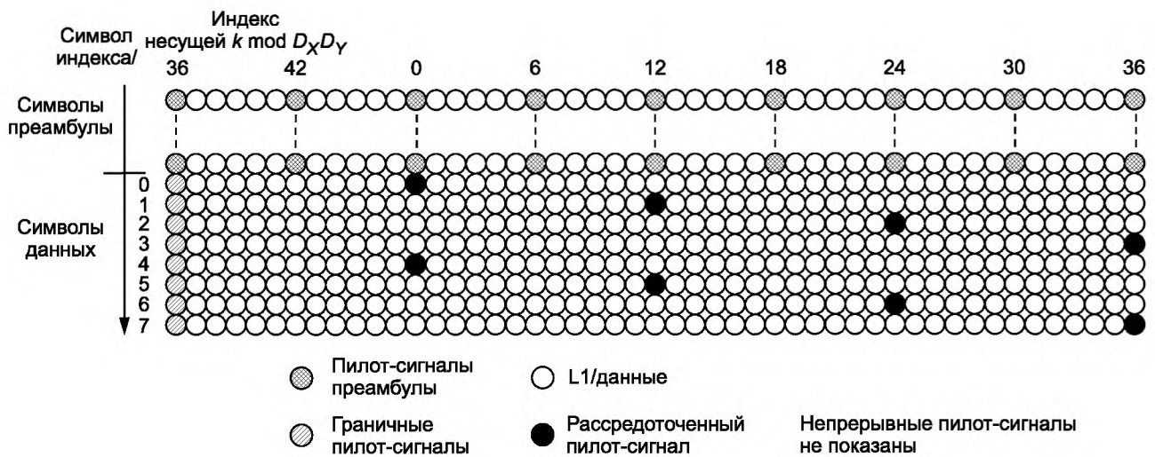
Рисунок Е.4 — Рассредоточенный пилот-сигнал для GI 1/64 с низкочастотной границей k \bmod D_x D_y = 36
