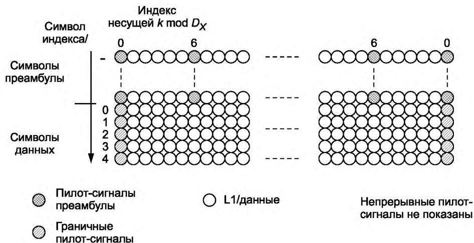
Рисунок 41 — Расположение граничных пилот-сигналов в спектре OFDM сигнала
