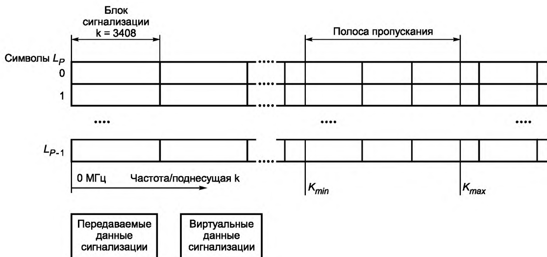
Рисунок 36 — Структура Символа Преамбулы в частотной области
