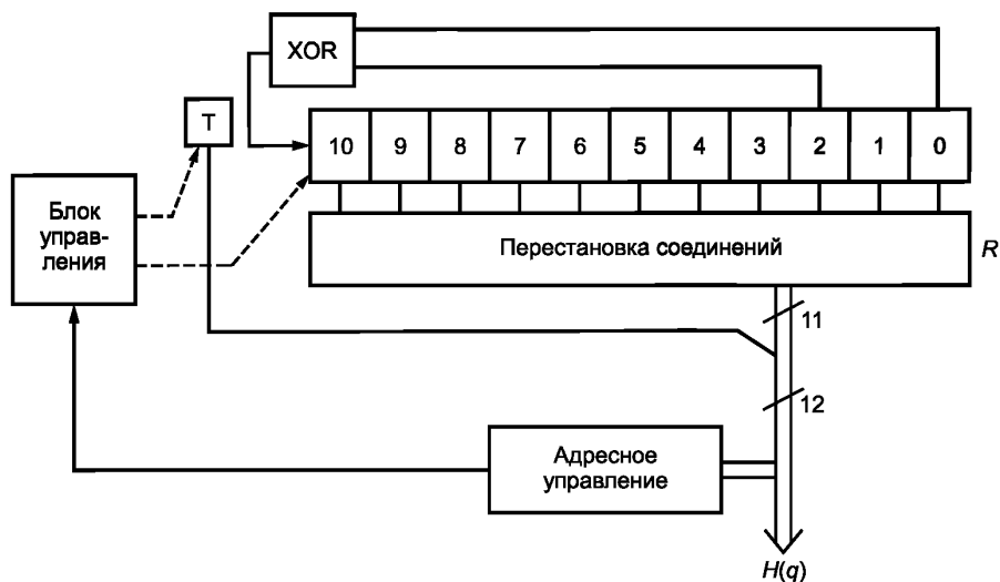
Рисунок 40 — Блок-схема алгоритма формирования функции перестановки перемежителя частоты режима 4К
