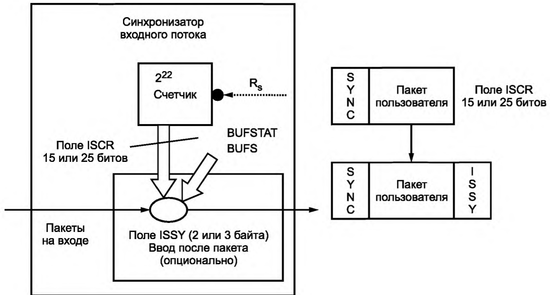
Рисунок А.1 – Блок-схема синхронизатора входного потока
