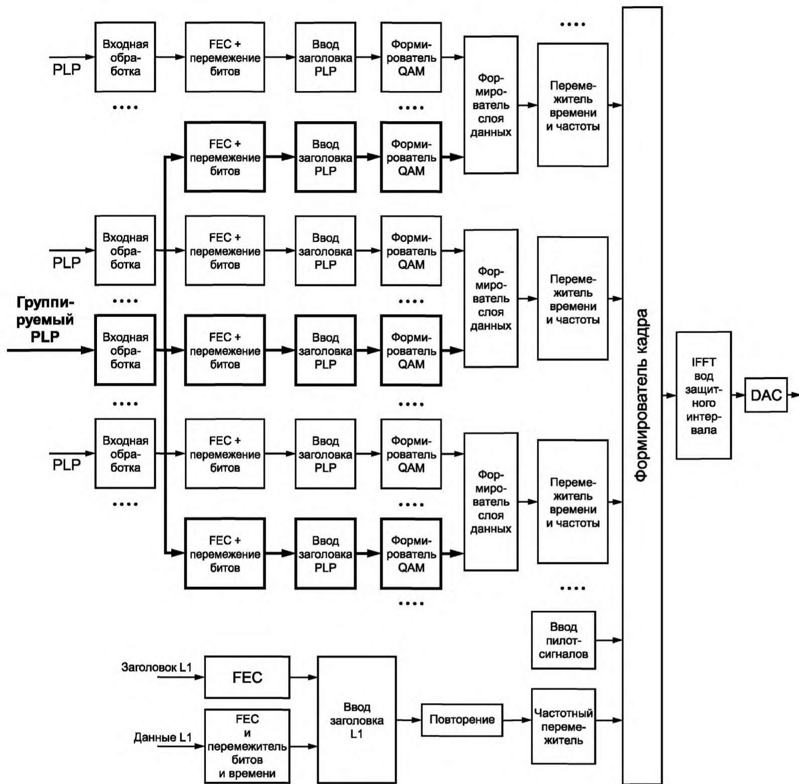
Рисунок Г.1 — Блок-схема режима группирования PLP
