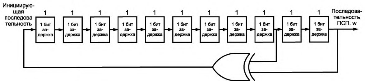
Рисунок 34 — Формирование псевдослучайной последовательности
