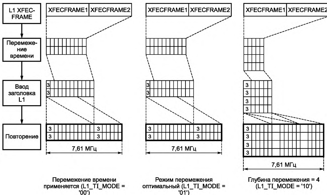
Рисунок 31 — Перемежевание времени данных сигнализации L1-part2
