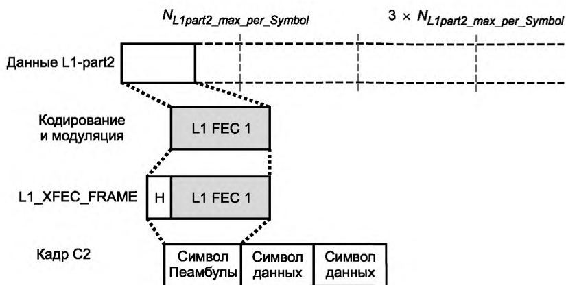
Рисунок 26 — Кодированные данные L1-part2
