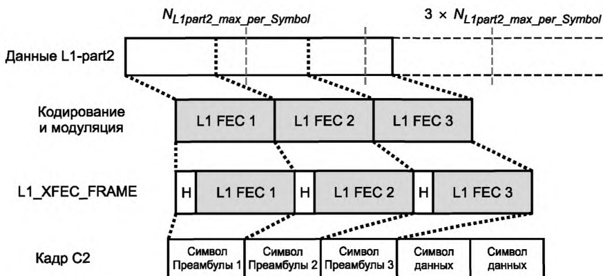
Рисунок 27 — Длина кодированных данных
