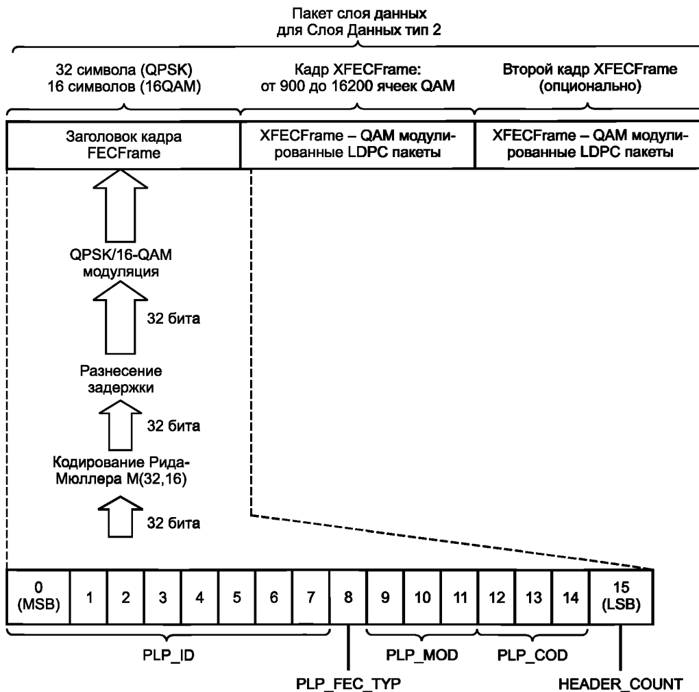
Рисунок 19 — Пакет Слоя Данных Тип 2, состоящий из заголовка FECFrame и следующих за ним пакетов XFECFrame
