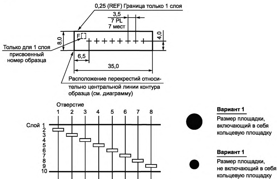
Рисунок В.8 — Тест-купон F
