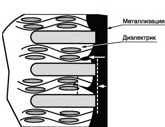
Рисунок 7 — Травление диэлектрика
