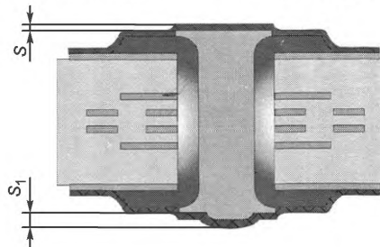
Рисунок 13 — Измерение толщины выступов «крышки»
