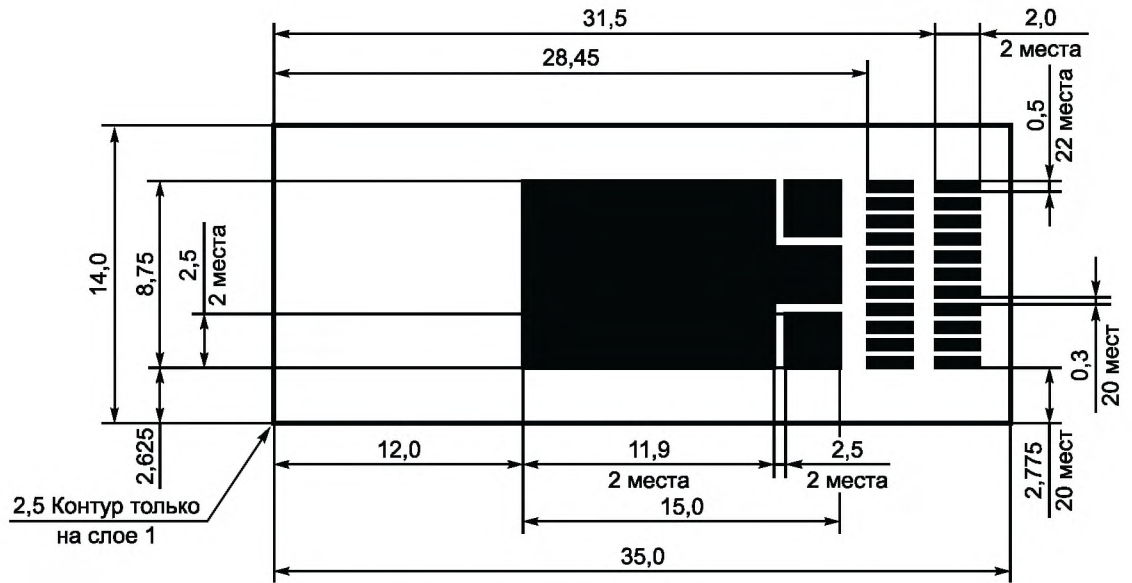
Рисунок В.12 — Тест-купон М
