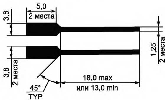
Рисунок В.3 — Тест-купон С
