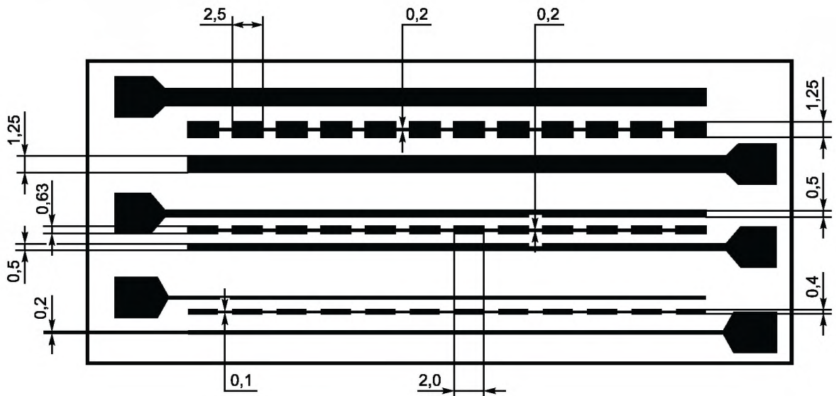
Рисунок В.13 — Тест-купон N
