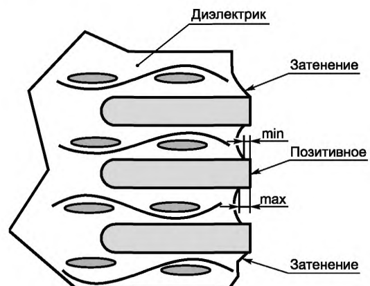
Рисунок 8 — Измерение значения травления диэлектрика
