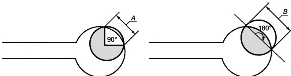
A = 1,414 \cdot радиус сквозного металлизированного отверстия; B — диаметр сквозного металлизированного отверстия
