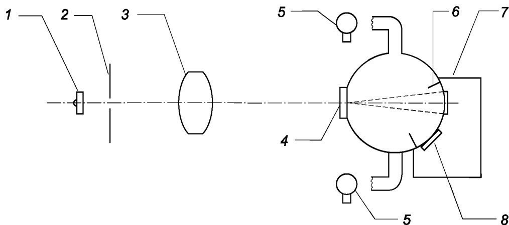
1 — фотодетектор; 2 — апертурная диафрагма; 3 — линза; 4 — образец; 5 — источник света; 6 — экран, 7 — световая ловушка; 8 — отражающий стандартный образец
