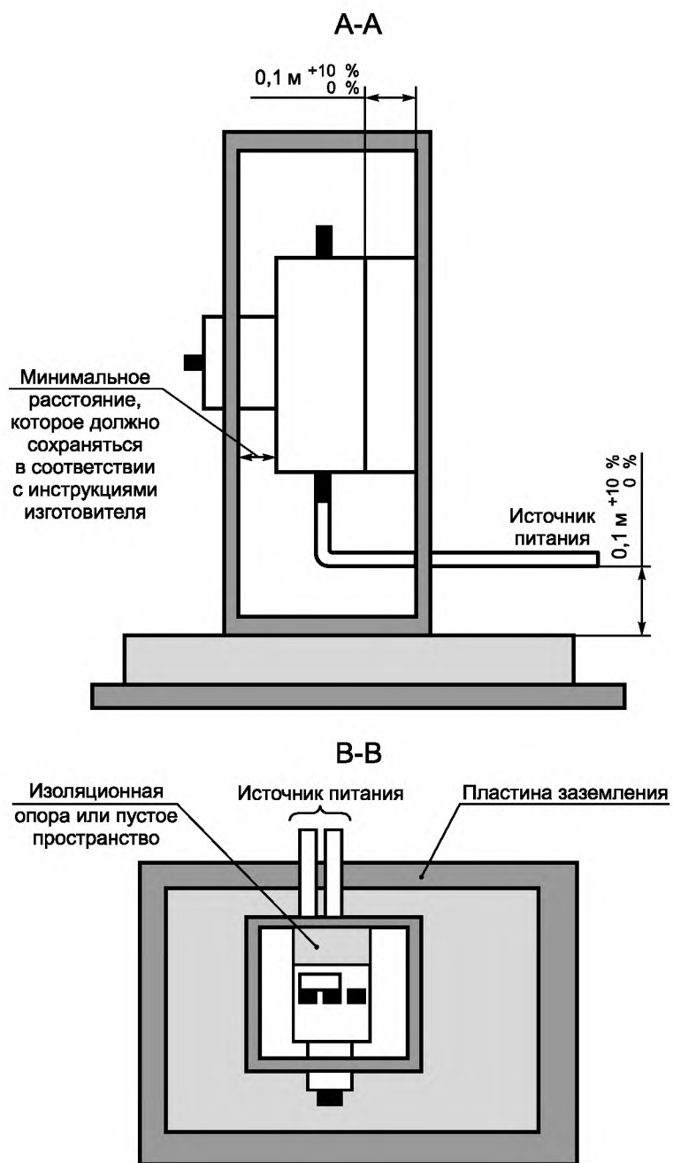
Рисунок 2b — Сечения А-А и В-В
