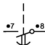
Замыкающий контакт с замедлением при замыкании
