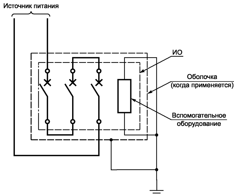
Рисунок 6 — Испытательная цепь для испытаний на излучение помех, устойчивость к гармоническим составляющим, провалам напряжения, электростатическим разрядам и электромагнитным полям. Трехфазная конфигурация с последовательным подключением полюсов
