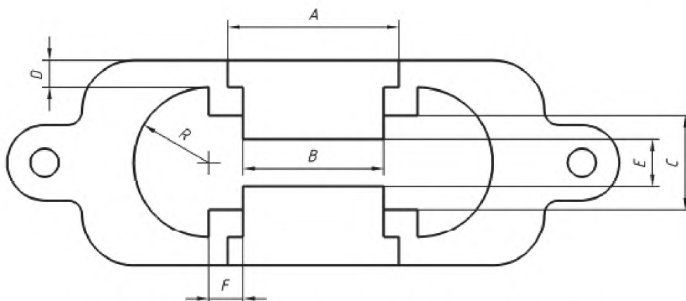
Рисунок 1 – Симметричная пресс-форма
