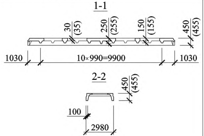
13 Плита типоразмера 2ПВ12 с четырьмя проемами размерами 1500×1700 мм
