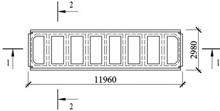
10 Плита типоразмера 2ПГ12
