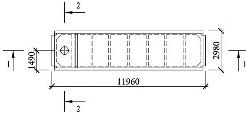
6 Плита типоразмера 1ПВ12 с проемом диаметром 1450 мм
