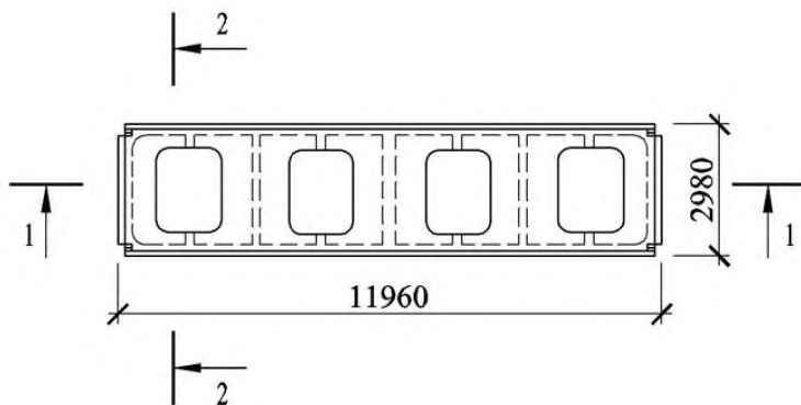
7 Плита типоразмера 1ПФ12 с четырьмя проемами размерами 1500×1700 мм
