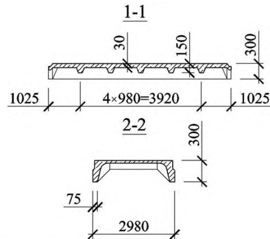
22 Плита типоразмера ЗПВ6 с проемами диаметром 400 или 700 мм
