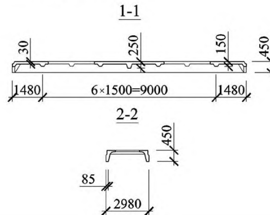
8 Плита типоразмера 1ПФ12 с двумя проемами размерами 2600×2700 мм
