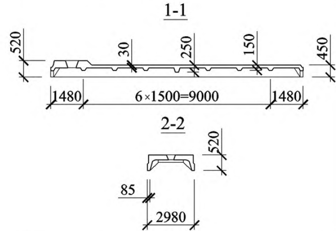
6 Плита типоразмера 1ПВ12 с проемом диаметром 1450 мм
