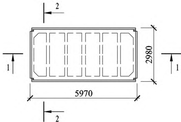
22 Плита типоразмера ЗПВ6 с проемами диаметром 400 или 700 мм
