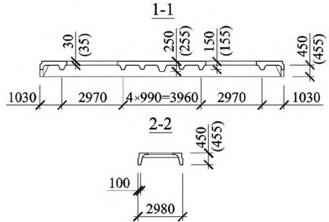
14 Плита типоразмера 2ПФ12 с двумя проемами размерами 2600×2700 мм
