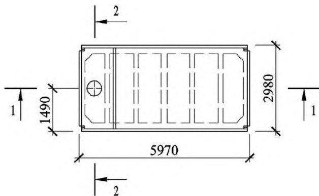
22 Плита типоразмера ЗПВ6 с проемами диаметром 400 или 700 мм
