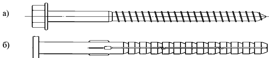
а) шуруп с шестигранной головкой с цилиндрическим буртом; б) дюбель с коническим входным отверстием
