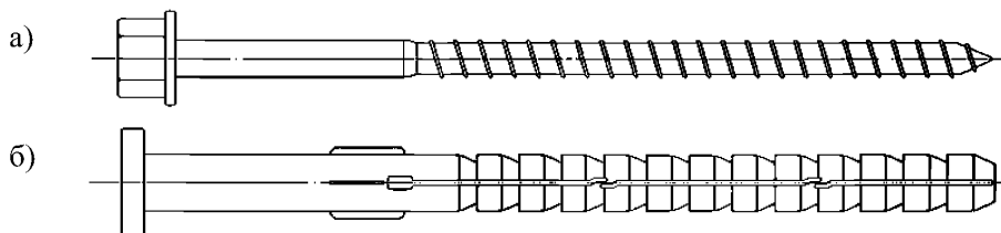
а) шуруп с шестигранной головкой с цилиндрическим буртом; б) дюбель с пресс-шайбой в месте входного отверстия
