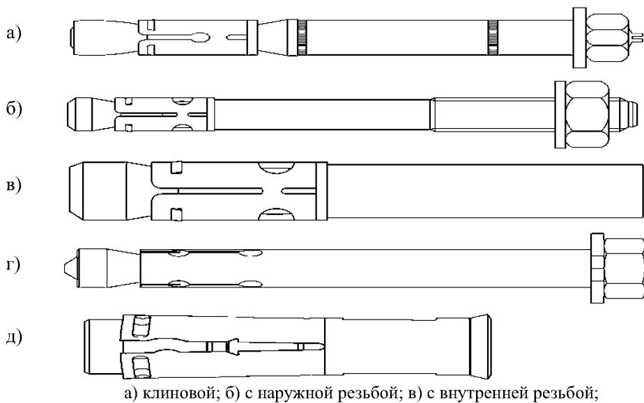
Рисунок А.6 – Анкеры с контролируемым моментом затяжки
