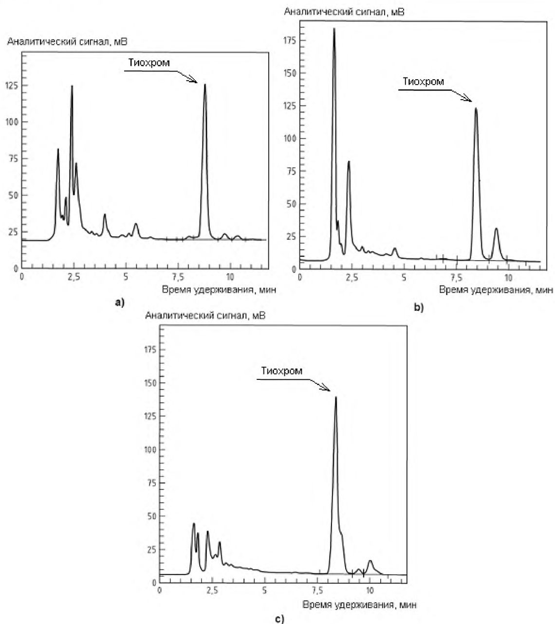
Рисунок В.2 — Примеры хроматограмм экстрактов проб салата (а), вареного риса (б) и вареной свинины (с) с добавлением градуировочного раствора тиамин с применением послеколоночной дериватизации
