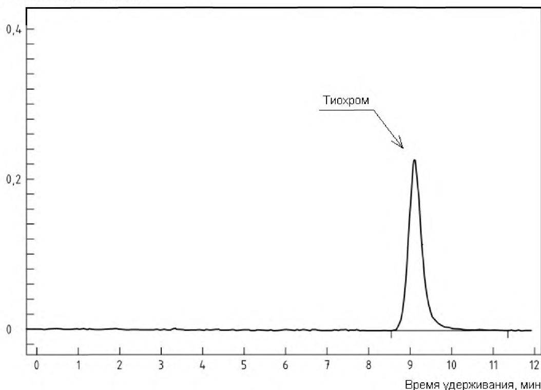
Рисунок В.1 — Пример хроматограммы градуировочного раствора тиамин с использованием предколоночной дериватизации с получением тиохрома
