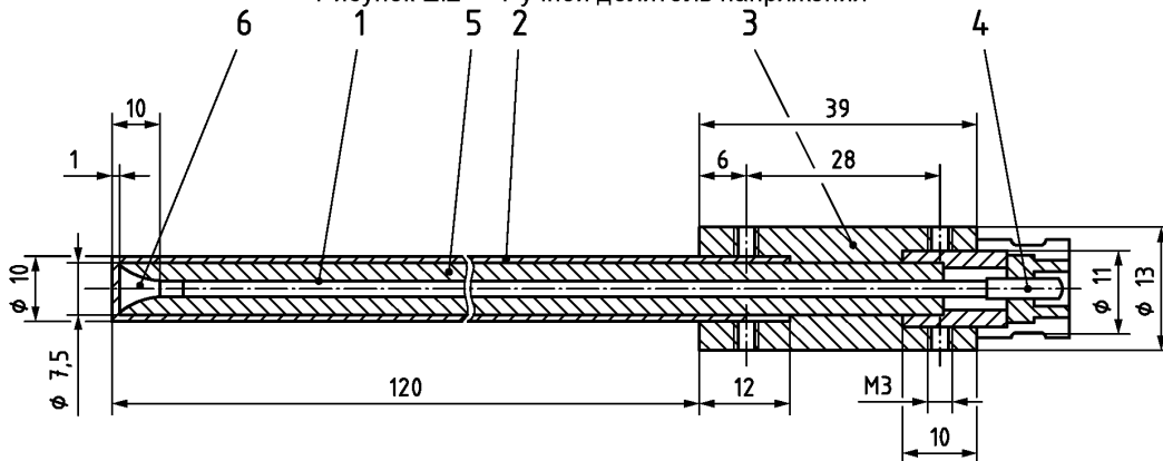
Рисунок Е.2 — Ручной делитель напряжения
