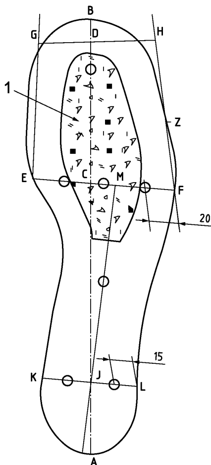
Рисунок А.1 — Рисунок несъемной стельки
