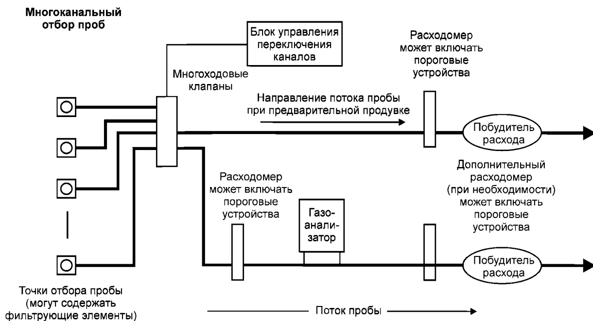
Рисунок А.2 — Типичные конфигурации пробоотборных линий
