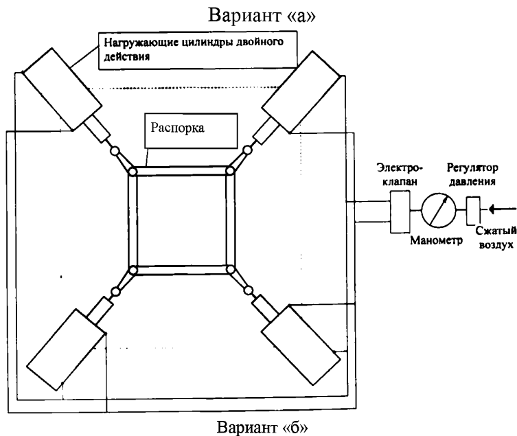
Рисунок 6. Схемы испытаний распорок дистанционных на ток имитируемого короткого замыкания. Вариант «а» и «б»
