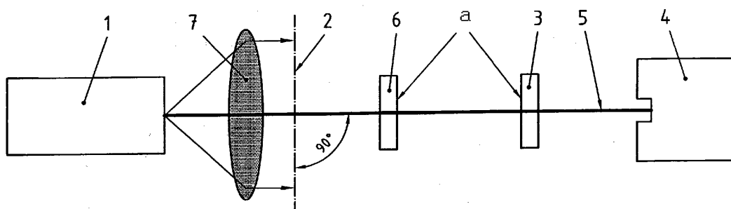
1 – лазер; 2 – опорная (референтная) ось; 3 – поляризатор; 4 – приемник излучения; 5 – лазерный пучок; 6 – четвертьволновая пластина; 7 – коллиматор; а – вращение в пределах 180^\circ
