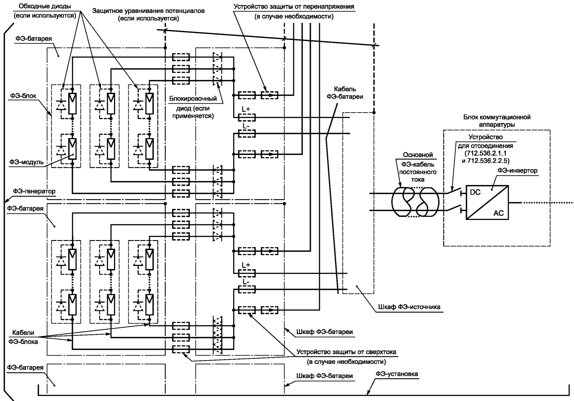
Рисунок 712.2 — ФЭ установка. Пример с несколькими батареями
