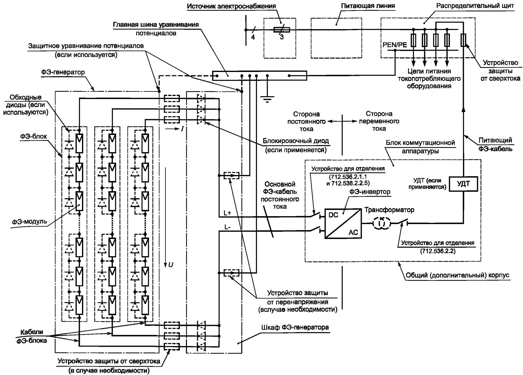
Рисунок 712.1 — ФЭ установка. Общая схема. Одна батарея
