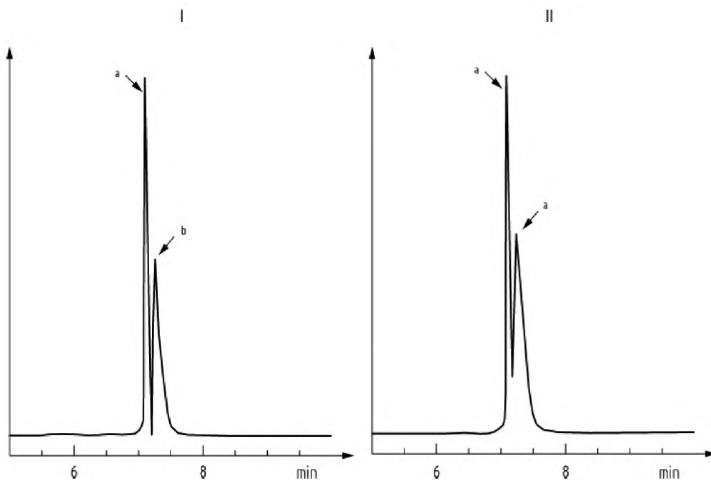
I - промышленный образец \text{Fe}^{3+} /EDDHSA; II - стандартный образец \text{Fe}^{3+} /EDDHSA; а и b - различные формы \text{Fe}^{3+} /EDDHSA
